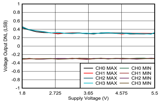
图 6-11. 电压输出 DNL 与电源电压间的关系
