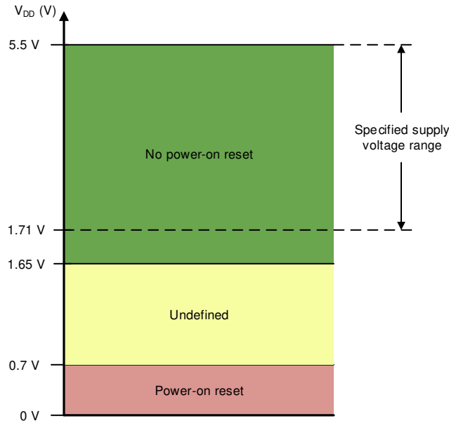
图 7-15. V_{DD} POR 电路的阈值电平
