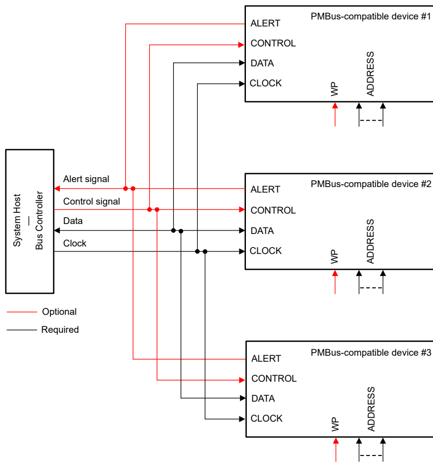
图 7-11. PMBus 连接
