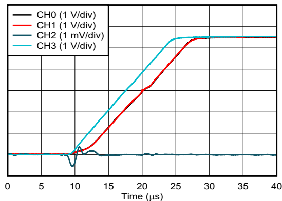
图 6-23. 电压输出上电干扰
