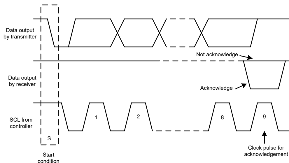
图 7-20. I 2 C 总线上的确认和非确认
