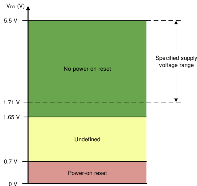
图 7-15. Threshold Levels for V_{DD} POR Circuit
