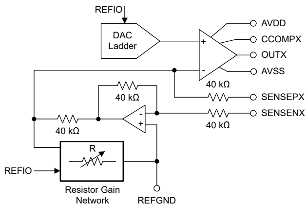
图 8-3. Voltage Output Buffer
