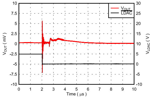
图 7-37. Glitch Impulse, 1 LSB Step, Falling Edge
