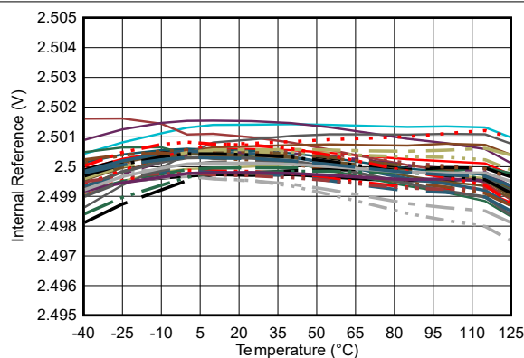
图 5-44. 内部基准电压与温度间的关系 (TSSOP)
