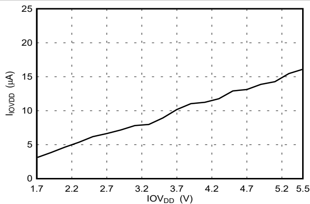
图 5-29. 电源电流 ( I_{\text{IOVDD}} ) 与电源电压间的关系
