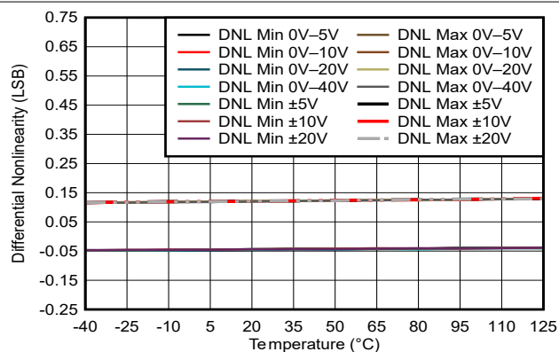
图 5-17. DAC81401 DNL 与温度间的关系
