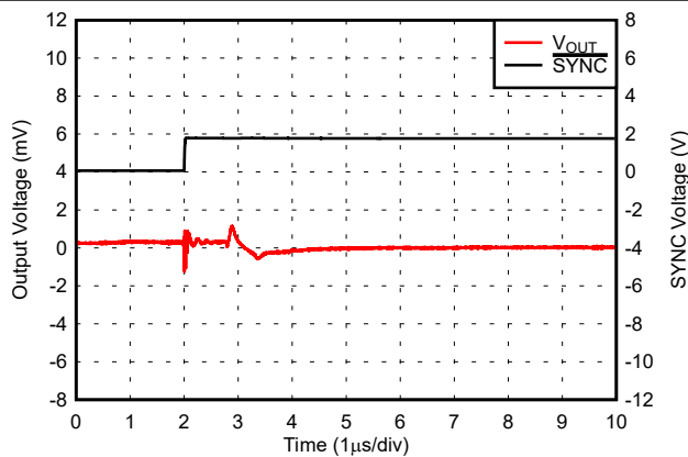
图 5-38. 干扰脉冲，1LSB 步长，下降沿
