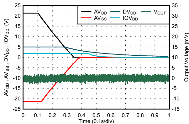
图 5-40. 关断响应
