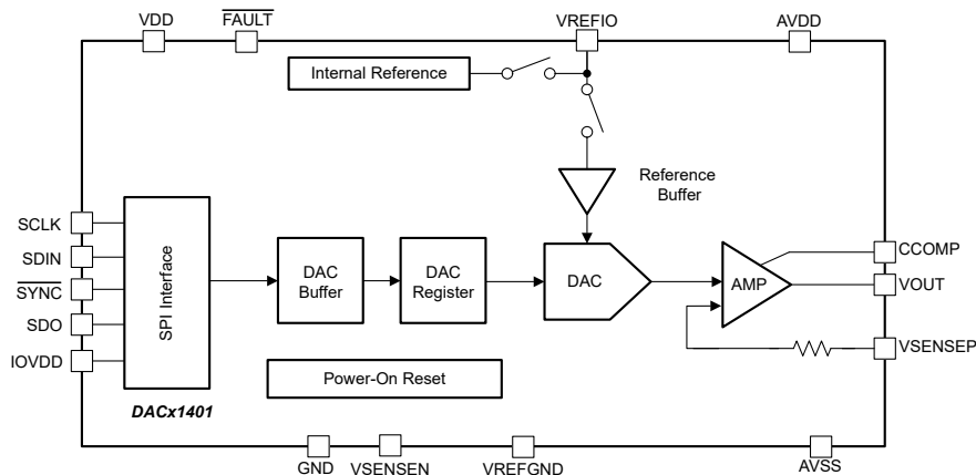
DACx1401 方框图
