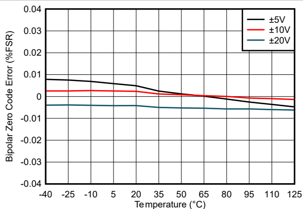
图 5-23. 双极零代码误差与温度间的关系
