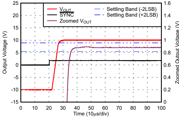
图 5-34. 满标度建立时间，上升沿
