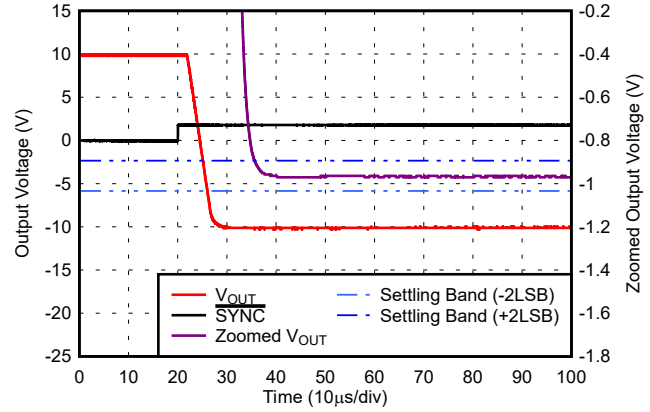
图 5-35. 满标度建立时间，下降沿
