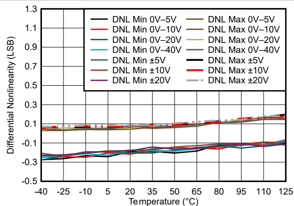
图 5-17. DAC81401 DNL 与温度间的关系
