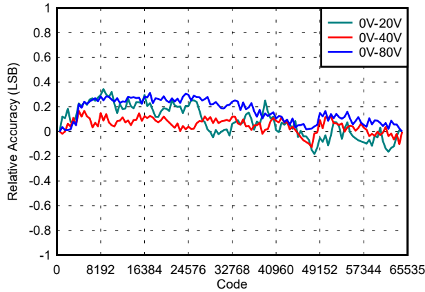
图 8-4. 相对精度与数字输入代码间的关系 (单极模式)
