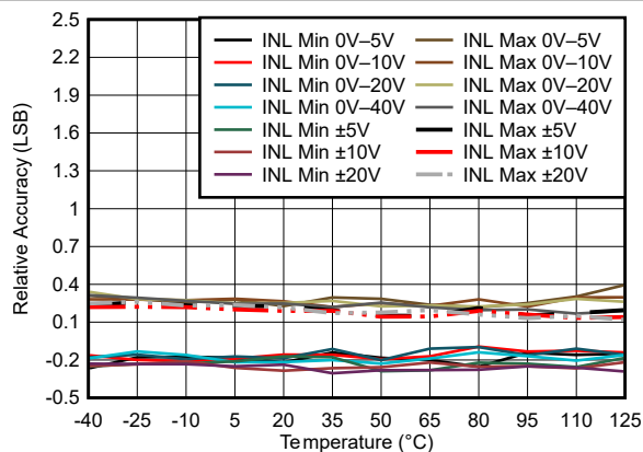
图 5-16. DAC81401 相对精度与温度间的关系
