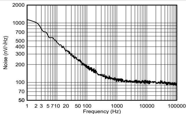
图 5-41. DAC 输出噪声密度与频率间的关系
