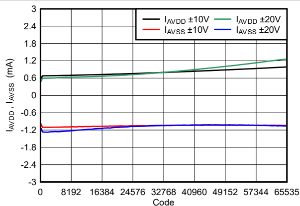
图 5-28. 电源电流 ( I_{\text{AVDD}} 、 I_{\text{AVSS}} ) 与数字输入代码间的关系
