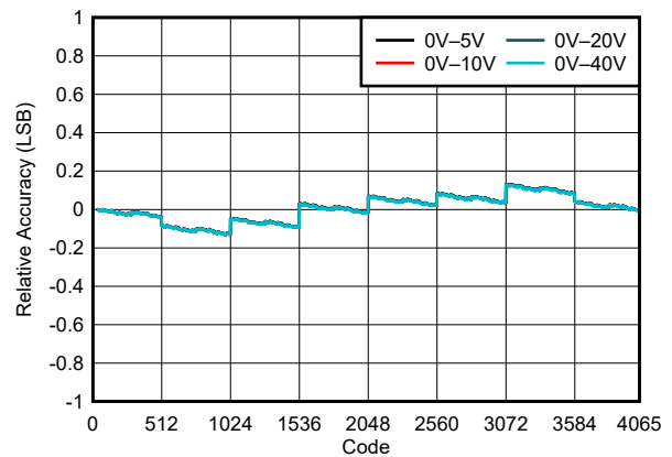
图 5-11. DAC61401 相对精度与数字输入代码间的关系 (单极输出)
