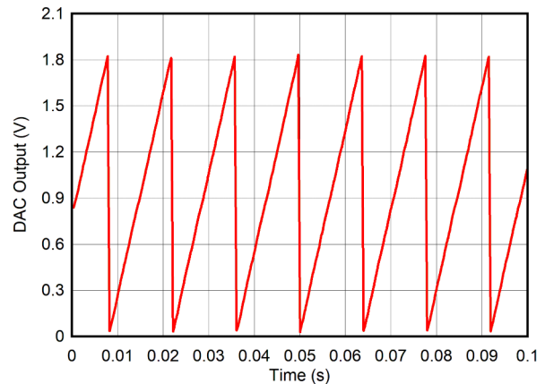
图 9-3. Sawtooth Waveform
