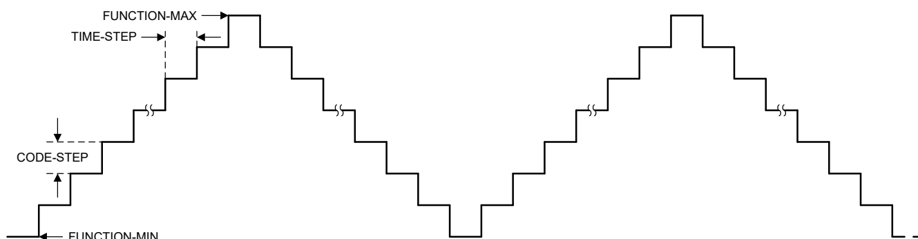
图 6-10. 三角波形
