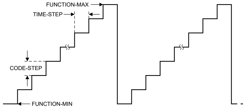
图 6-11. 锯齿波形
