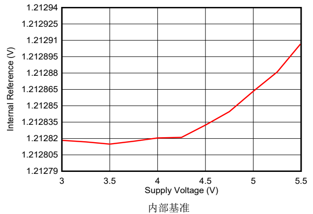
图 5-54. 内部基准与电源电压间的关系
