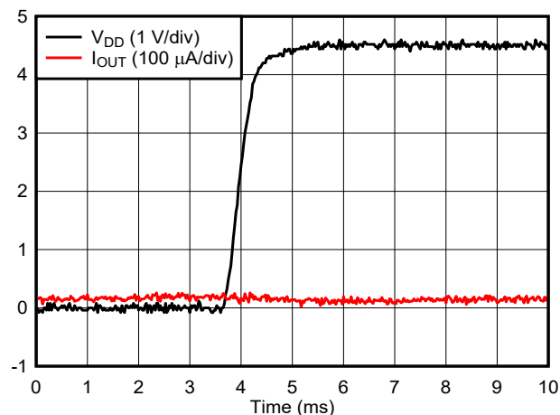
图 5-42. 电流输出上电干扰
