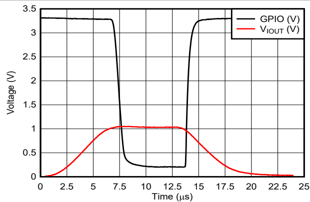
图 8-3. 比较器切换
