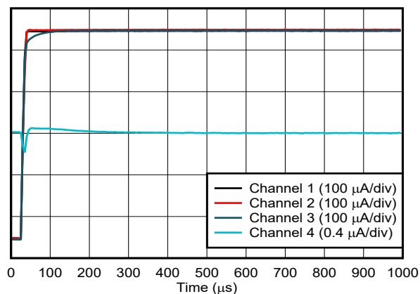
图 6-45. 电流输出上电干扰
