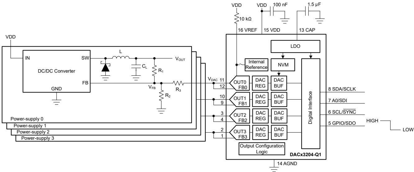
图 8-1. APD 偏置
