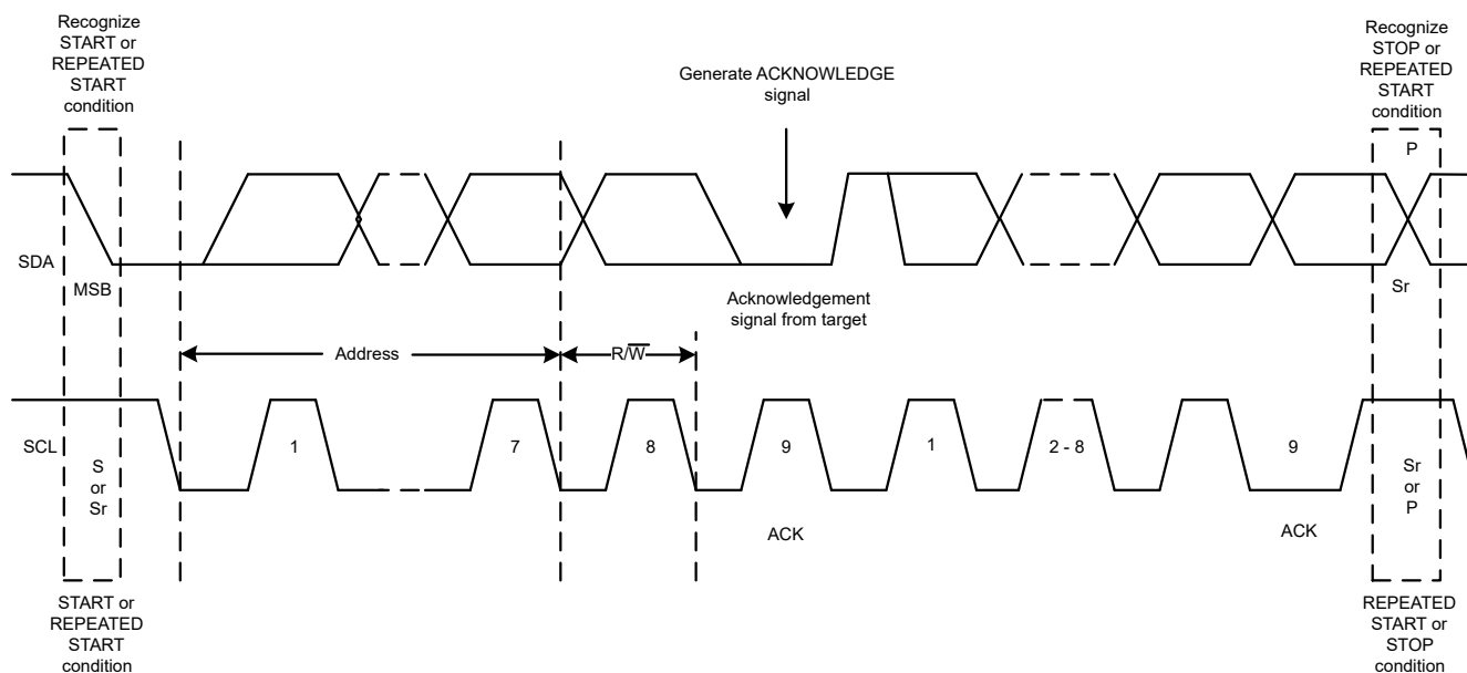
图 7-23. I 2 C 总线协议
