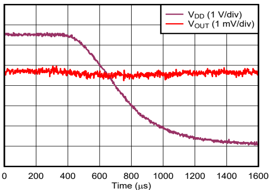
图 6-22. 电压输出建立时间 - 下降沿
