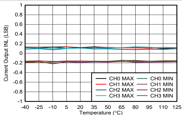
图 6-32. 电流输出 INL 与温度间的关系
