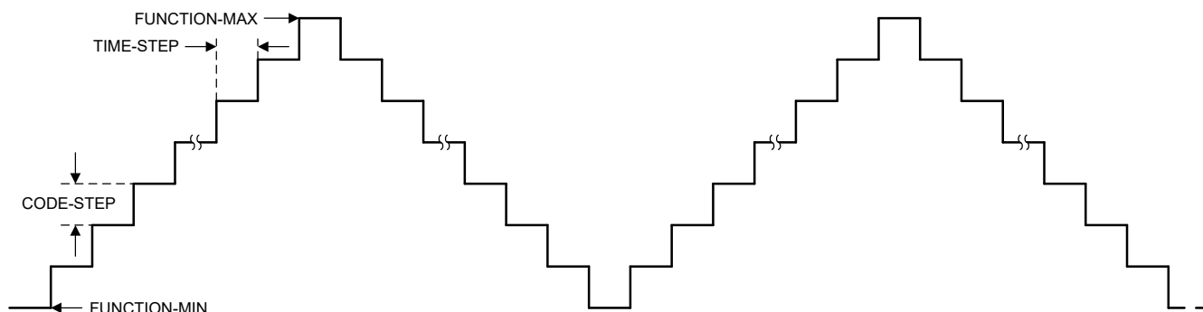
图 7-12. 三角波形
