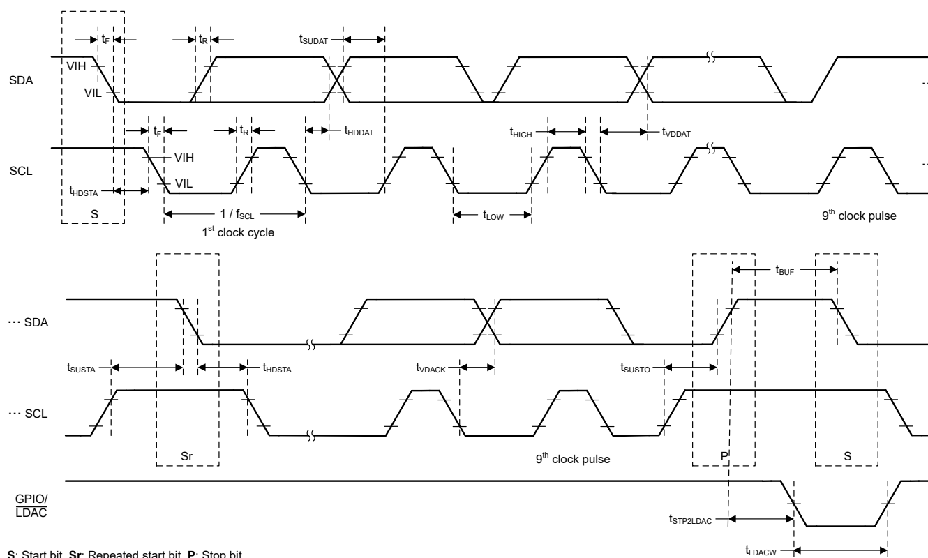
图 6-1. I 2 C 时序图
