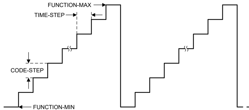
图 7-13. 锯齿波形
