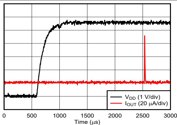
图 6-43. 电流输出建立时间 (上升沿)
