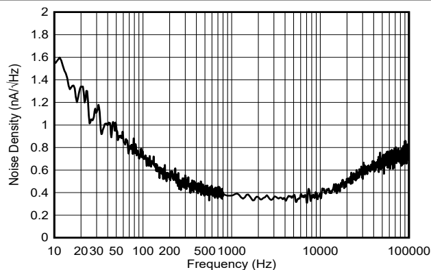
图 6-49. 电流输出噪声密度
