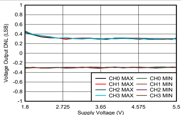
图 6-11. 电压输出 DNL 与电源电压间的关系
