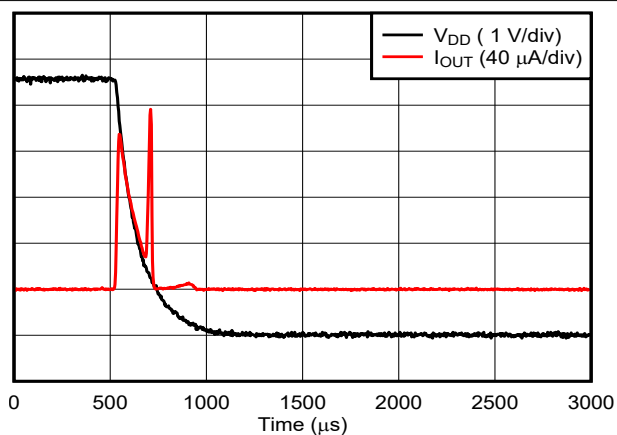
图 6-44. 电流输出建立时间 (下降沿)
