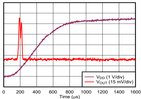
图 6-23. 电压输出上电干扰
