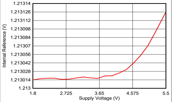
图 6-55. 内部基准与电源电压间的关系
