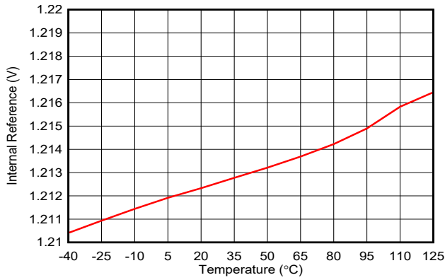
图 6-54. 内部基准与温度间的关系
