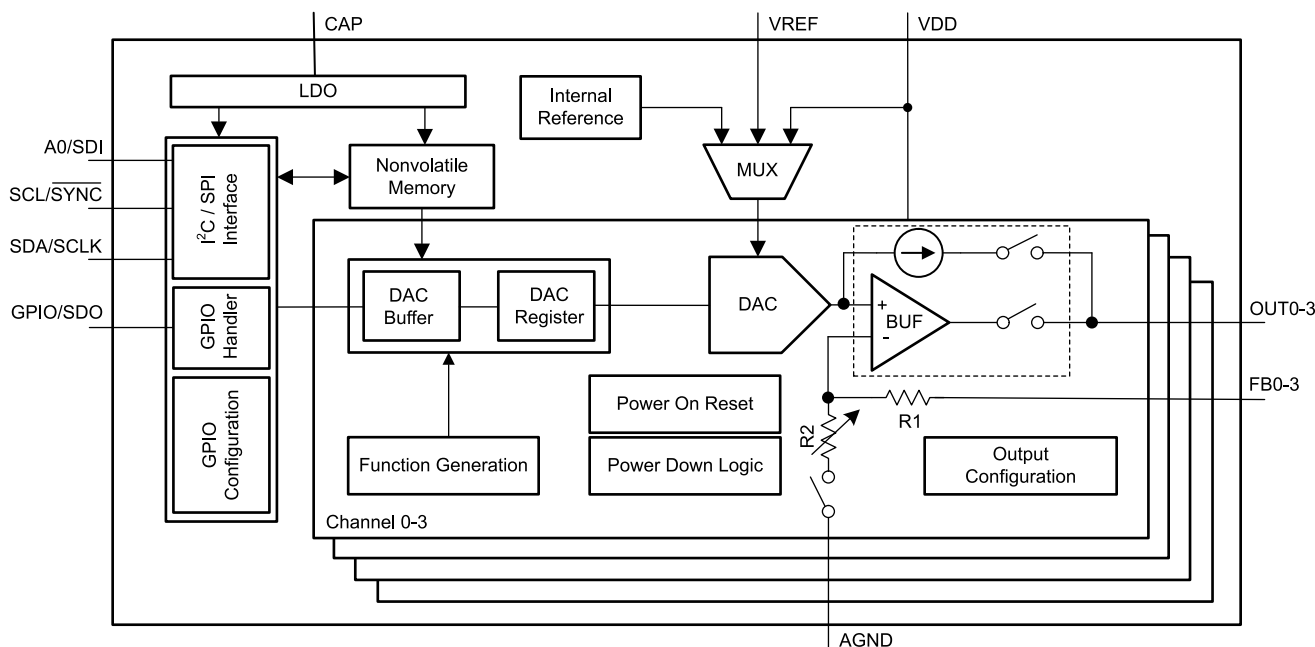
图 7-1. 功能方框图
