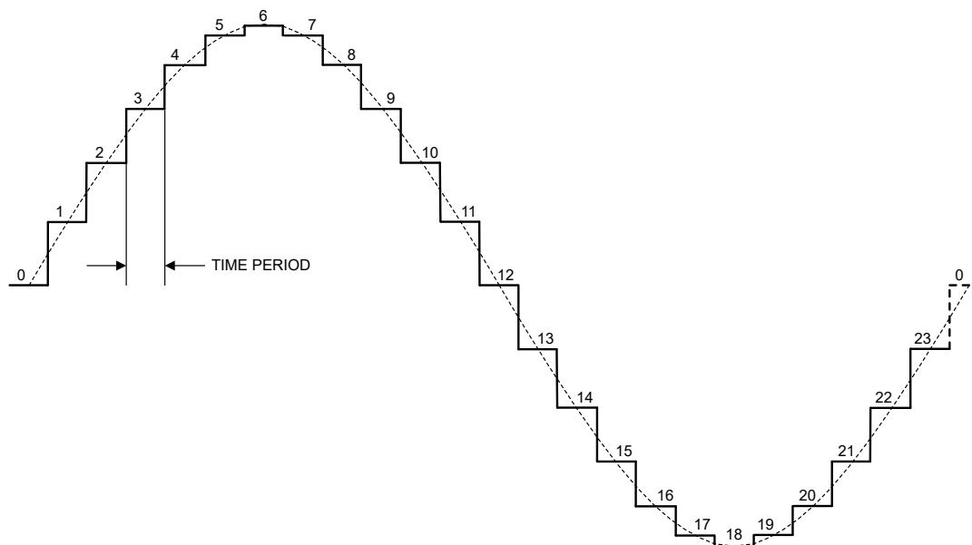
图 7-14. 正弦波生成
