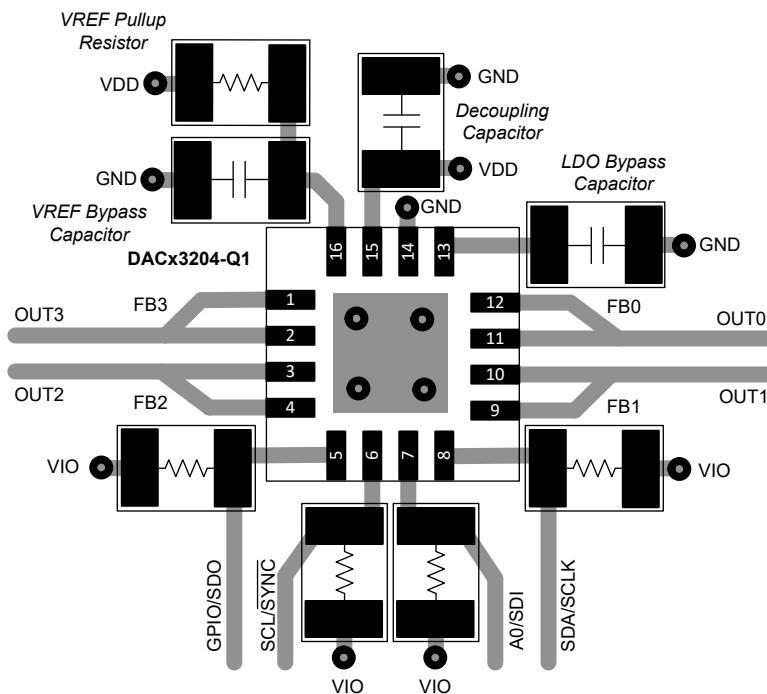
图 8-4. 布局示例
