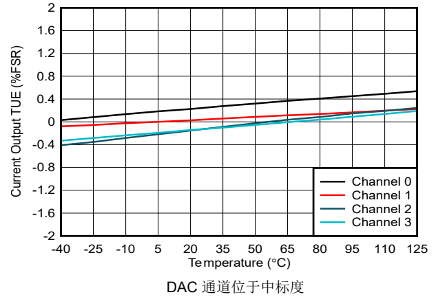
图 5-44. 电流输出 TUE 与温度间的关系
