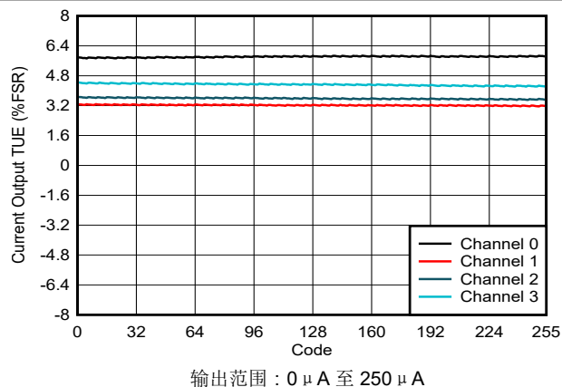
图 5-42. 电流输出 TUE 与数字输入代码间的关系
