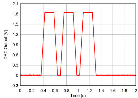
图 9-9. Medium Priority Alarm
