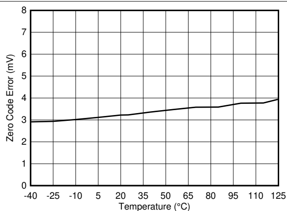
图 7-7. Zero Code Error vs Temperature
