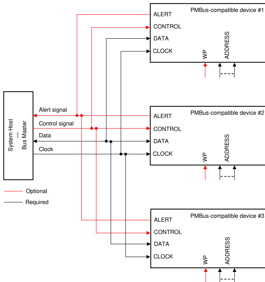
图 8-2. PMBus Connections
