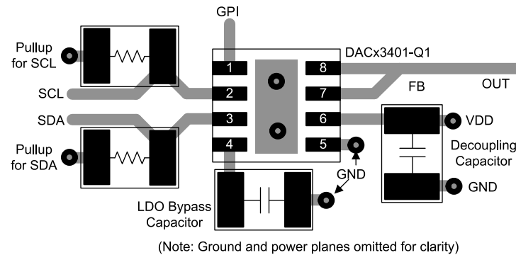
图 11-1. Layout Example
