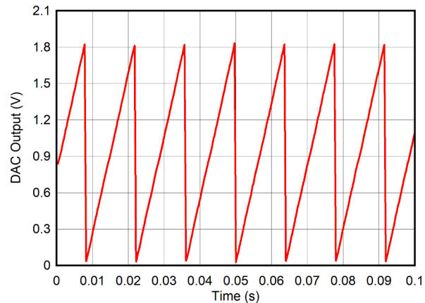
图 9-3. Sawtooth Waveform
