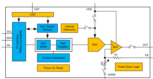
功能方框图
