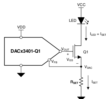
使用 DACx3401-Q1 的 LED 偏置
