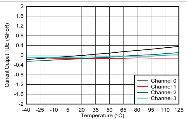
图 6-38. 电流输出 TUE 与温度间的关系
