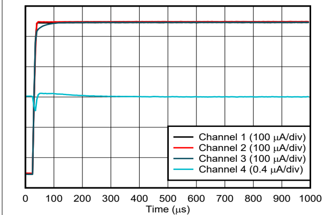
图 6-45. 电流输出加电干扰
