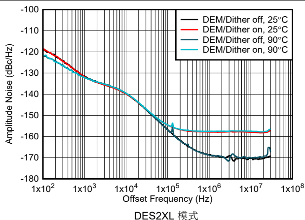
图 6-202. 1GHz 条件下振幅噪声与偏移频率和温度间的关系
