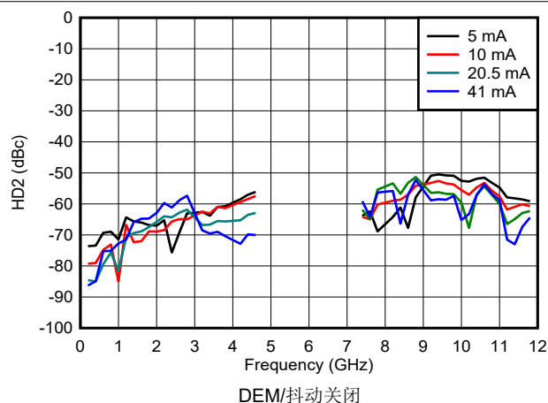
图 6-136. DES2X 模式下 HD2 与频率和输出电流间的关系
