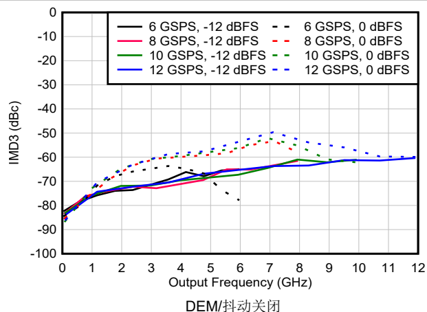
图 6-125. DES2X 模式下 IMD3 与频率和采样速率间的关系
