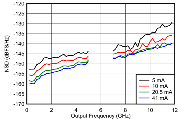
图 6-61. NSD 与输出频率和输出电流间的关系
