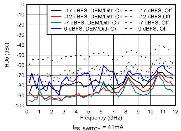
图 6-179. NRZ/RF 模式下 HD5 与频率和数字振幅间的关系
