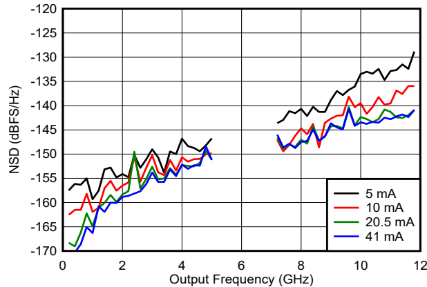
图 6-60. NSD 与输出频率和输出电流间的关系
