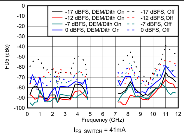
图 6-181. DES2X 模式下 HD5 与频率和数字振幅间的关系
