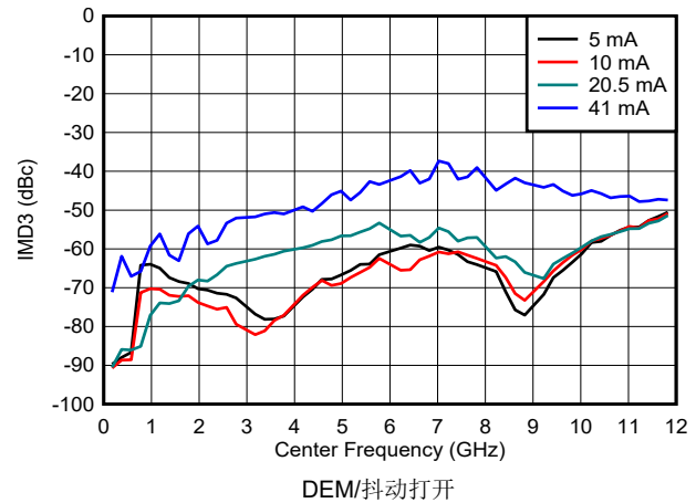
图 6-107. NRZ/RF 模式下 IMD3 与频率和输出电流间的关系
