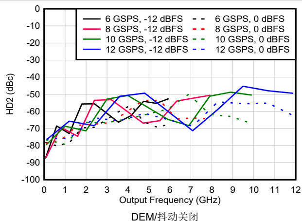
图 6-149. DES2X 模式下 HD2 与频率和采样速率间的关系
