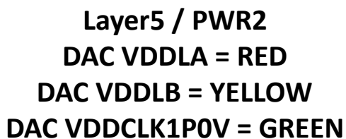
图 8-31. 第 5 层的电源平面布局
