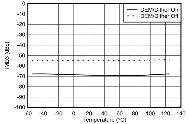
图 6-129. 9002MHz DES2XH 模式下 IMD3 与温度间的关系
