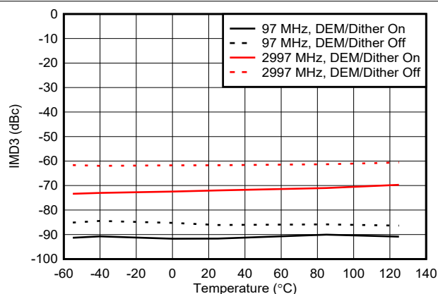
图 6-126. NRZ 模式下 IMD3 与温度间的关系
