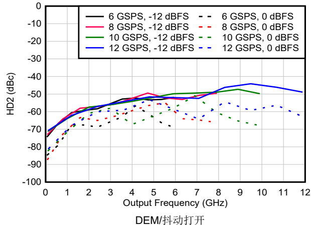
图 6-146. NRZ/RF 模式下 HD2 与频率和采样速率间的关系
