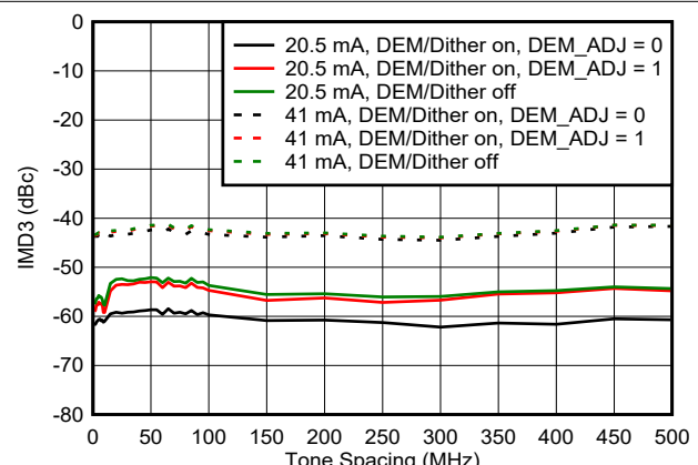
图 6-119. DES2XL 模式下 IMD3 与频率间隔间的关系
