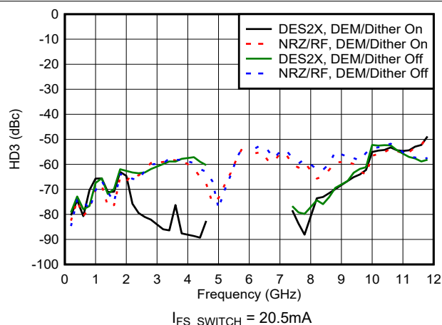
图 6-88. HD3 与频率和模式间的关系
