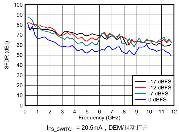
图 6-95. NRZ/RF 模式下 SFDR 与频率和数字振幅间的关系
