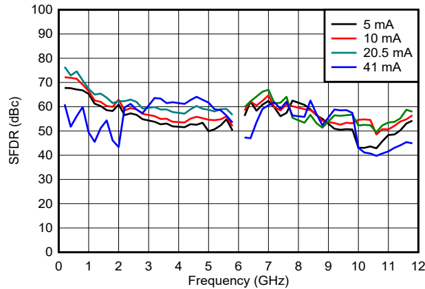
图 6-92. DES2X 模式下 SFDR 与频率和输出电流间的关系
