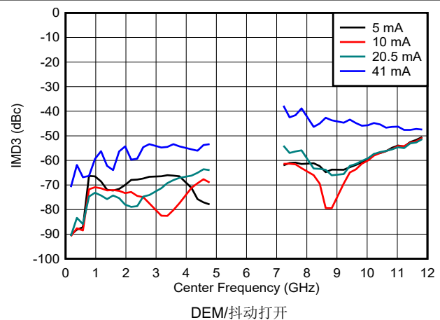
图 6-109. DES2X 模式下 IMD3 与频率和输出电流间的关系
