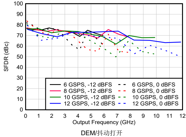
图 6-104. DES2X 模式下 SFDR 与频率和采样速率间的关系
