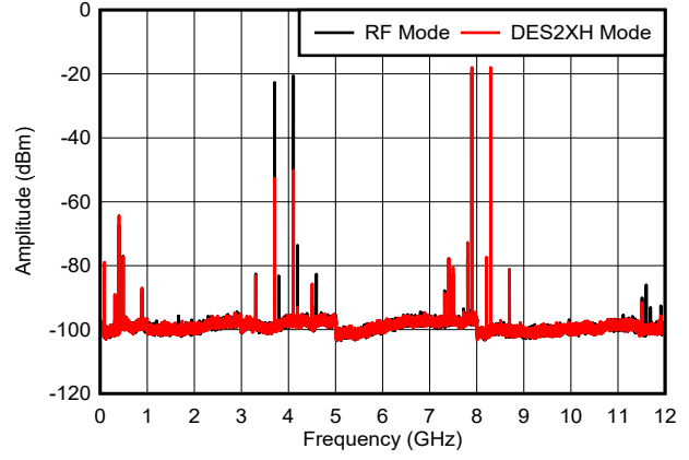
图 6-52. 双音， f_{\text{OUT}} = 8097\text{MHz} ，0dBFS
