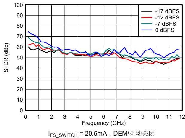
图 6-94. NRZ/RF 模式下 SFDR 与频率和数字振幅间的关系
