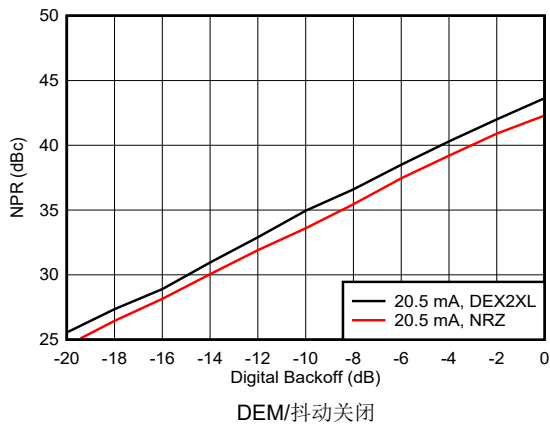
图 6-189. 噪声功率比与数字退避：第二个奈奎斯特区域
