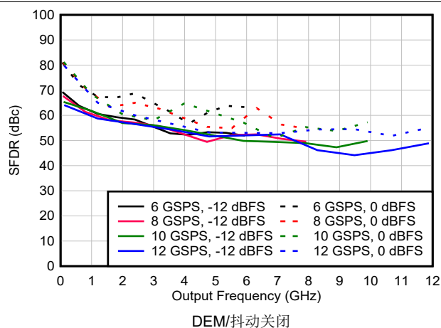
图 6-103. NRZ/RF 模式下 SFDR 与频率和采样速率间的关系
