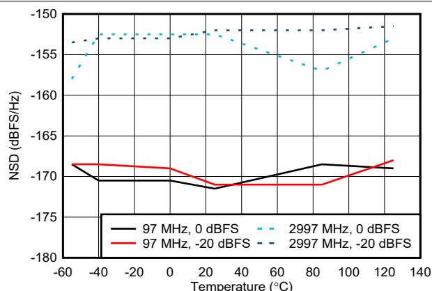
图 6-76. NSD 与温度间的关系
