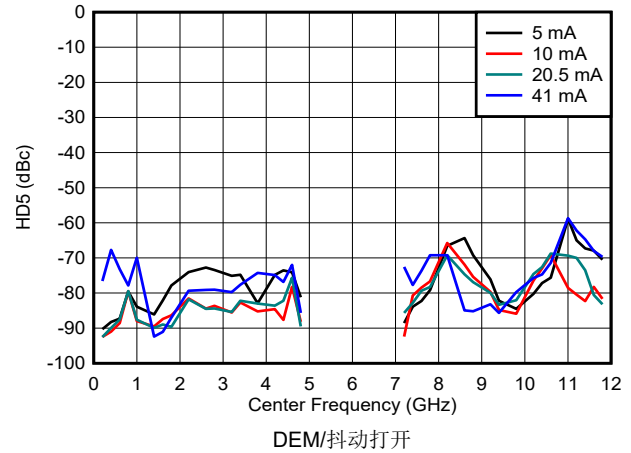
图 6-177. DES2X 模式下 HD5 与频率和输出电流间的关系
