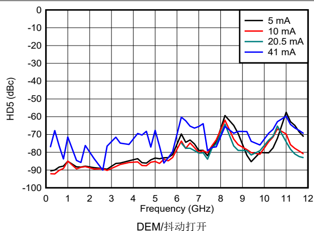
图 6-175. NRZ/RF 模式下 HD5 与频率和输出电流间的关系
