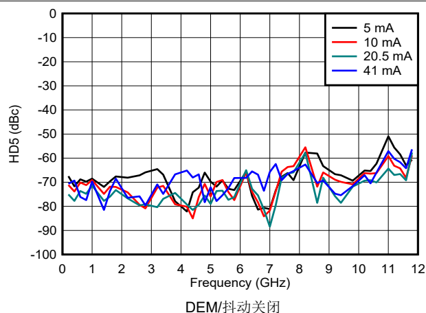
图 6-174. NRZ/RF 模式下 HD5 与频率和输出电流间的关系
