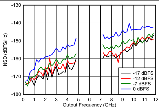
图 6-67. NSD 与输出频率和数字振幅间的关系
