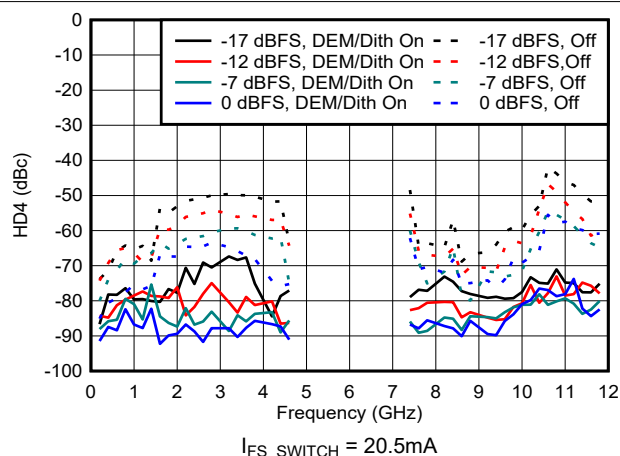
图 6-172. NRZ/RF 模式下 HD4 与频率和数字振幅间的关系
