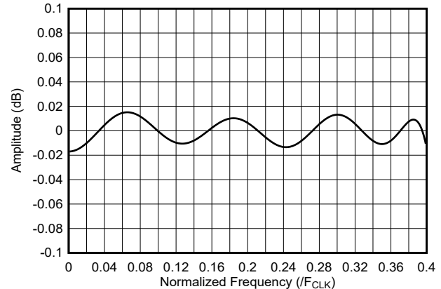
图 7-49. DES 内插器频率响应 (通带)
