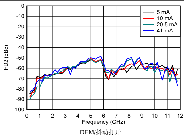
图 6-135. NRZ/RF 模式下 HD2 与频率和输出电流间的关系
