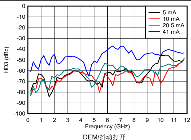
图 6-151. NRZ/RF 模式下 HD3 与频率和输出电流间的关系
