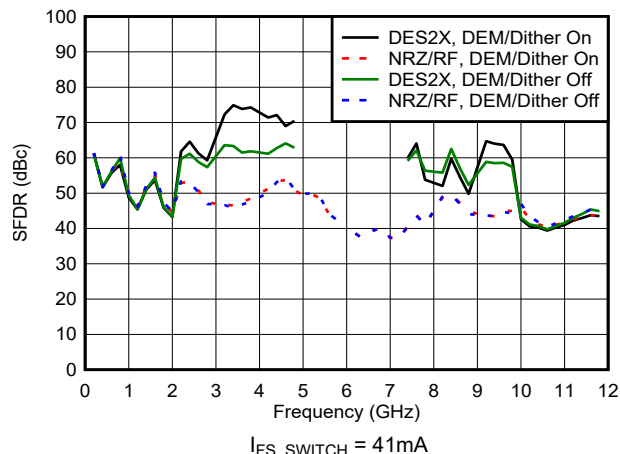
图 6-83. SFDR 与频率和模式间的关系
