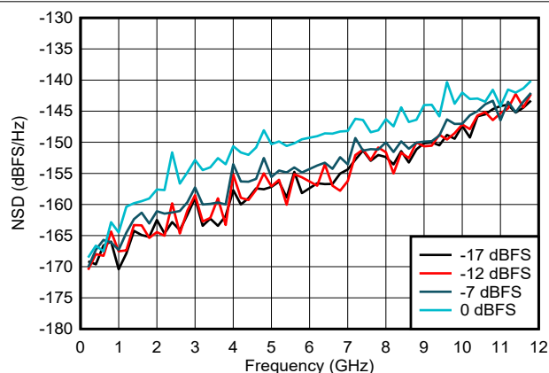
图 6-64. NSD 与输出频率和数字振幅间的关系
