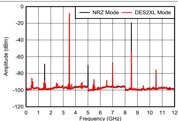
图 6-26. f_{\text{OUT}} = 2097\text{MHz} ，-6dBFS
