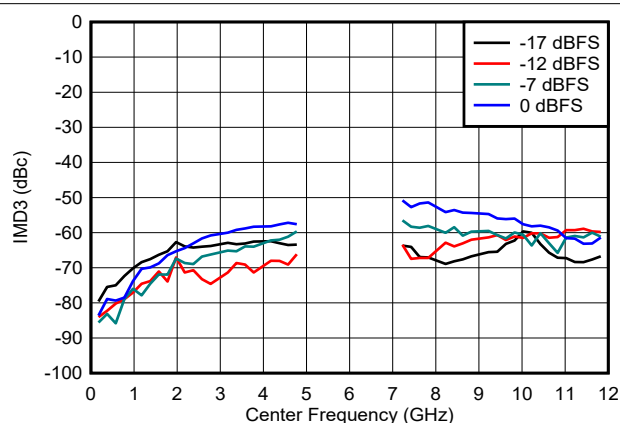
图 6-112. NRZ/RF 模式下 IMD3 与频率和数字振幅间的关系
