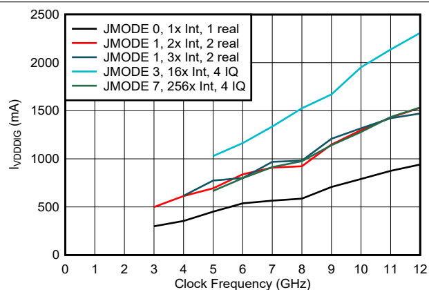
图 6-216. VDDDIG 电流与时钟频率和数字模式间的关系
