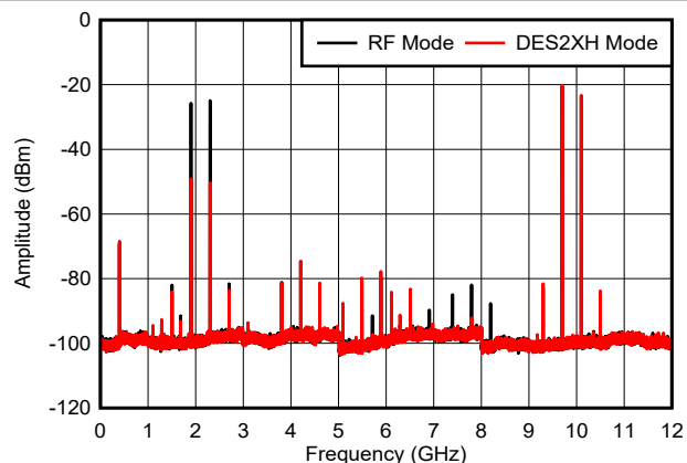
图 6-55. 双音， f_{\text{OUT}} = 9897\text{MHz} ，0dBFS
