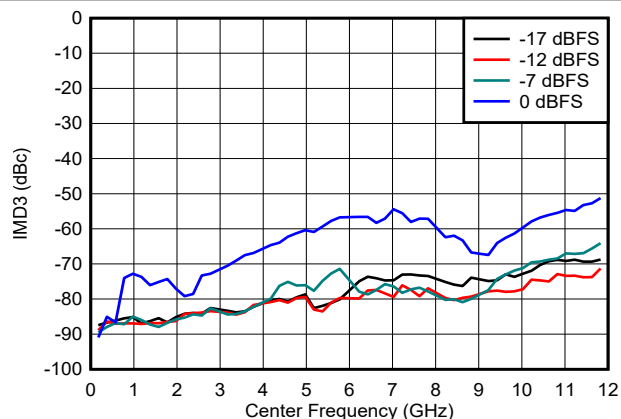
图 6-111. NRZ/RF 模式下 IMD3 与频率和数字振幅间的关系
