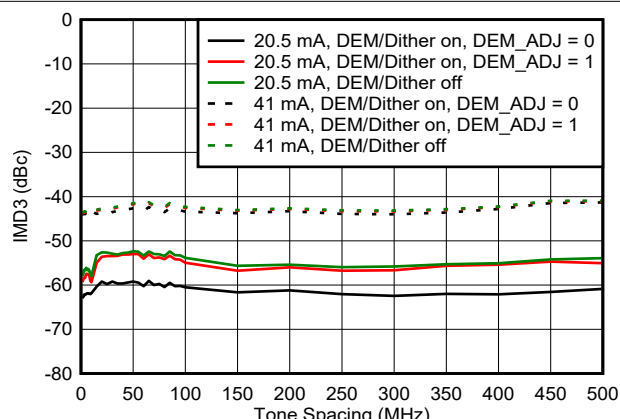
图 6-118. NRZ 模式下 IMD3 与频率间隔间的关系
