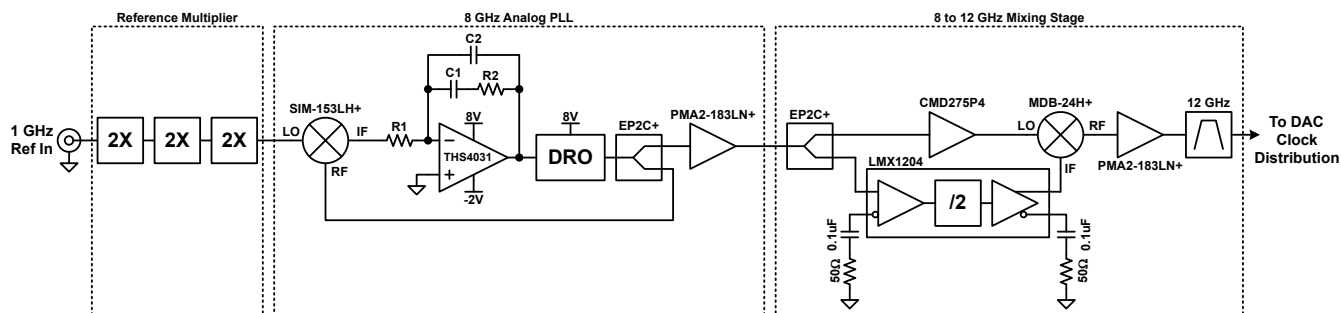
图 8-11. 12GHz 时钟合成器
