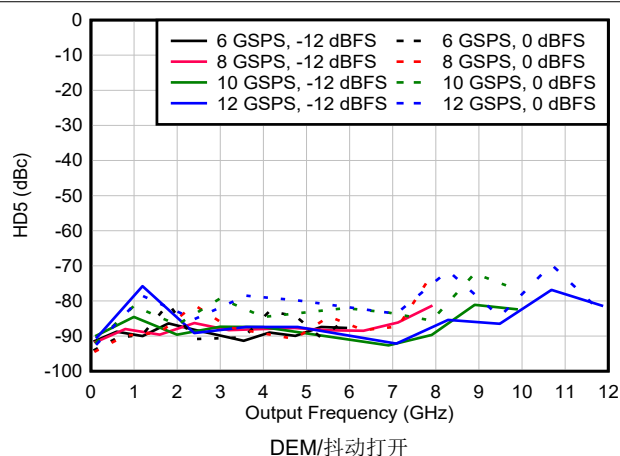
图 6-184. DES2X 模式下 HD5 与频率和采样速率间的关系
