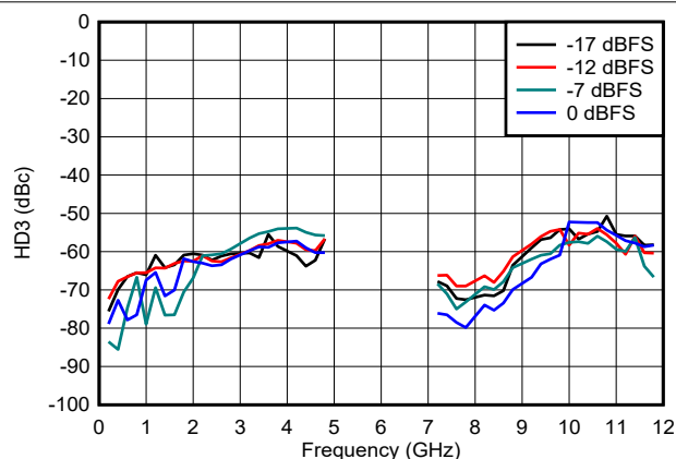
图 6-158. DES2X 模式下 HD3 与频率和数字振幅间的关系
