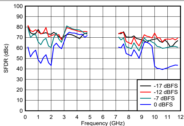
图 6-99. DES2X 模式下 SFDR 与频率和数字振幅间的关系
