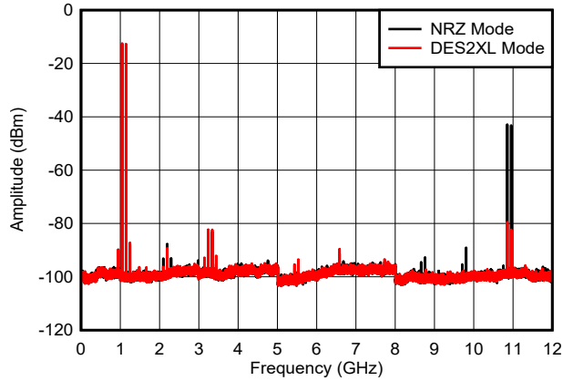
图 6-43. 双音， f_{\text{OUT}} = 1097\text{MHz} ，0dBFS
