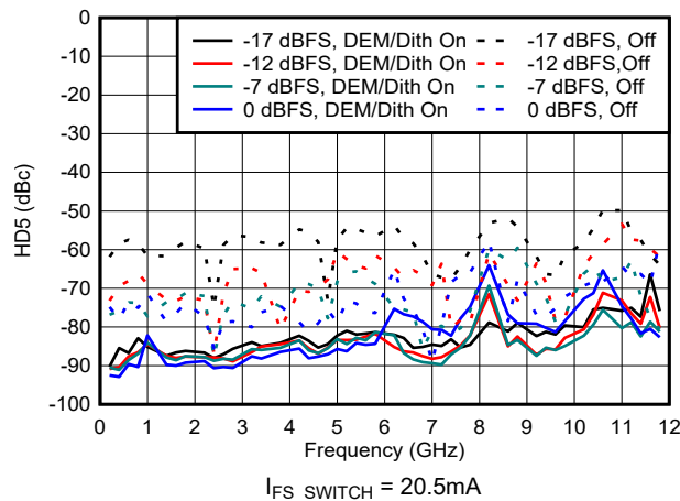
图 6-178. NRZ/RF 模式下 HD5 与频率和数字振幅间的关系
