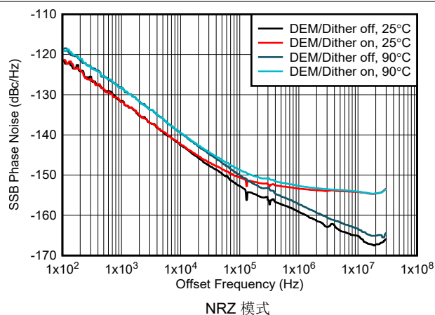
图 6-196. 1GHz 条件下相位噪声与偏移频率间的关系
