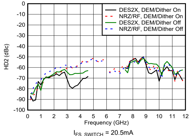
图 6-86. HD2 与频率和模式间的关系
