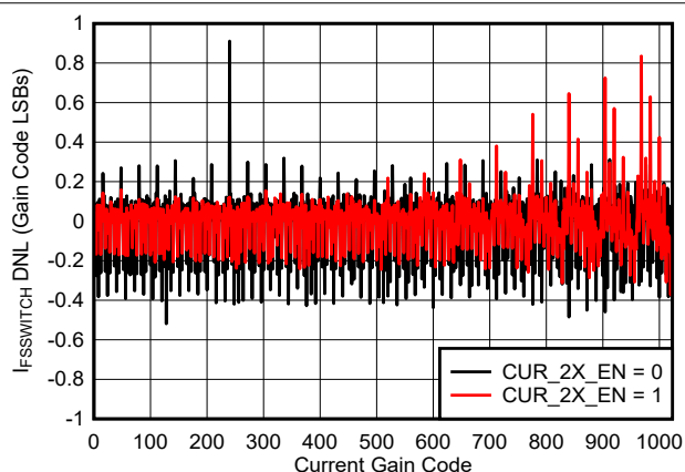
图 6-18. I_{\text{FS\_SWITCH}} 误差差分非线性与增益代码间的关系
