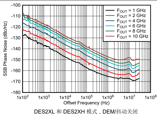
图 6-195. 相位噪声与偏移频率和输出频率间的关系
