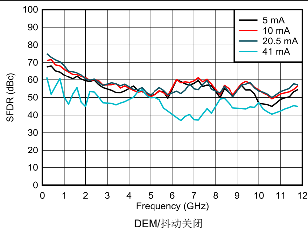
图 6-90. NRZ/RF 模式下 SFDR 与频率和输出电流间的关系
