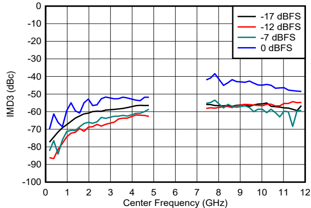
图 6-116. DES2X 模式下 IMD3 与频率和数字振幅间的关系
