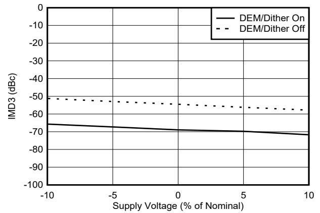
图 6-133. 9002MHz DES2XH 模式下 IMD3 与电压间的关系
