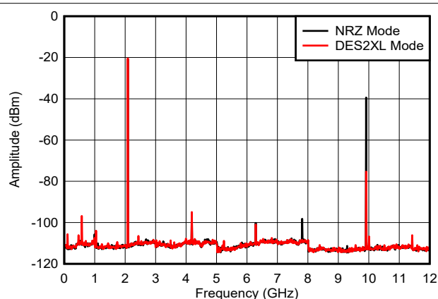
图 6-25. f_{\text{OUT}} = 2097\text{MHz} ，0dBFS
