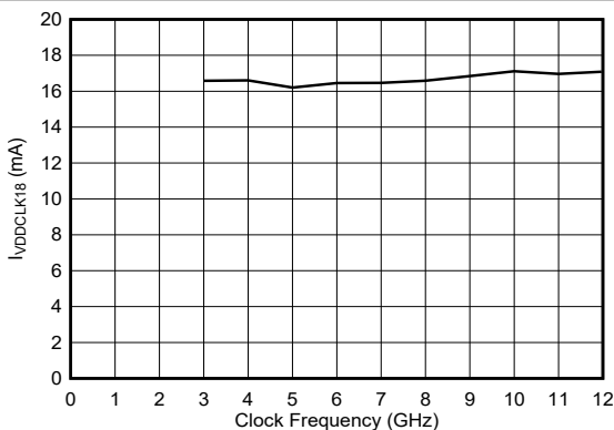
图 6-209. VDDCLK18 电流与时钟频率间的关系
