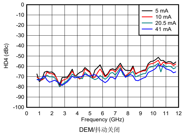
图 6-166. NRZ/RF 模式下 HD4 与频率和输出电流间的关系
