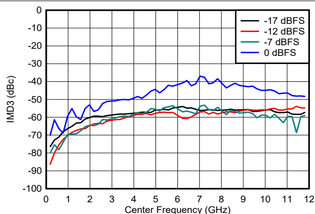
图 6-110. NRZ/RF 模式下 IMD3 与频率和数字振幅间的关系
