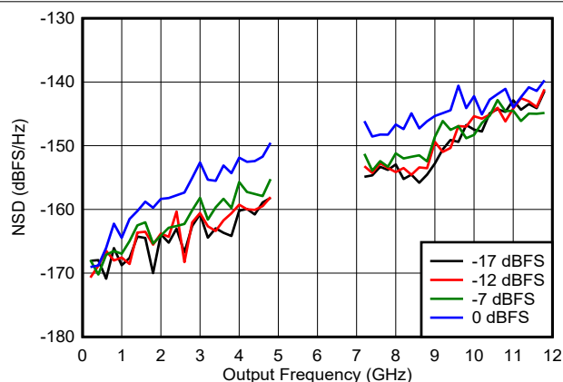
图 6-66. NSD 与输出频率和数字振幅间的关系
