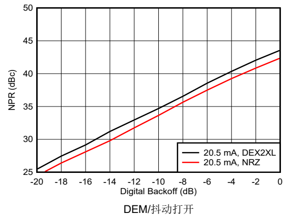
图 6-190. 噪声功率比与数字退避：第二个奈奎斯特区域
