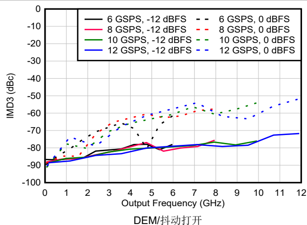
图 6-122. NRZ/RF 模式下 IMD3 与频率和采样速率间的关系
