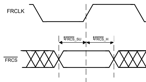
图 6-7. \overline{FRCS} 时序图
