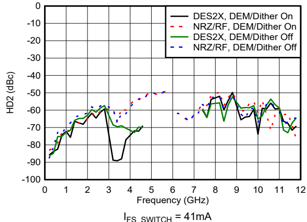
图 6-87. HD2 与频率和模式间的关系
