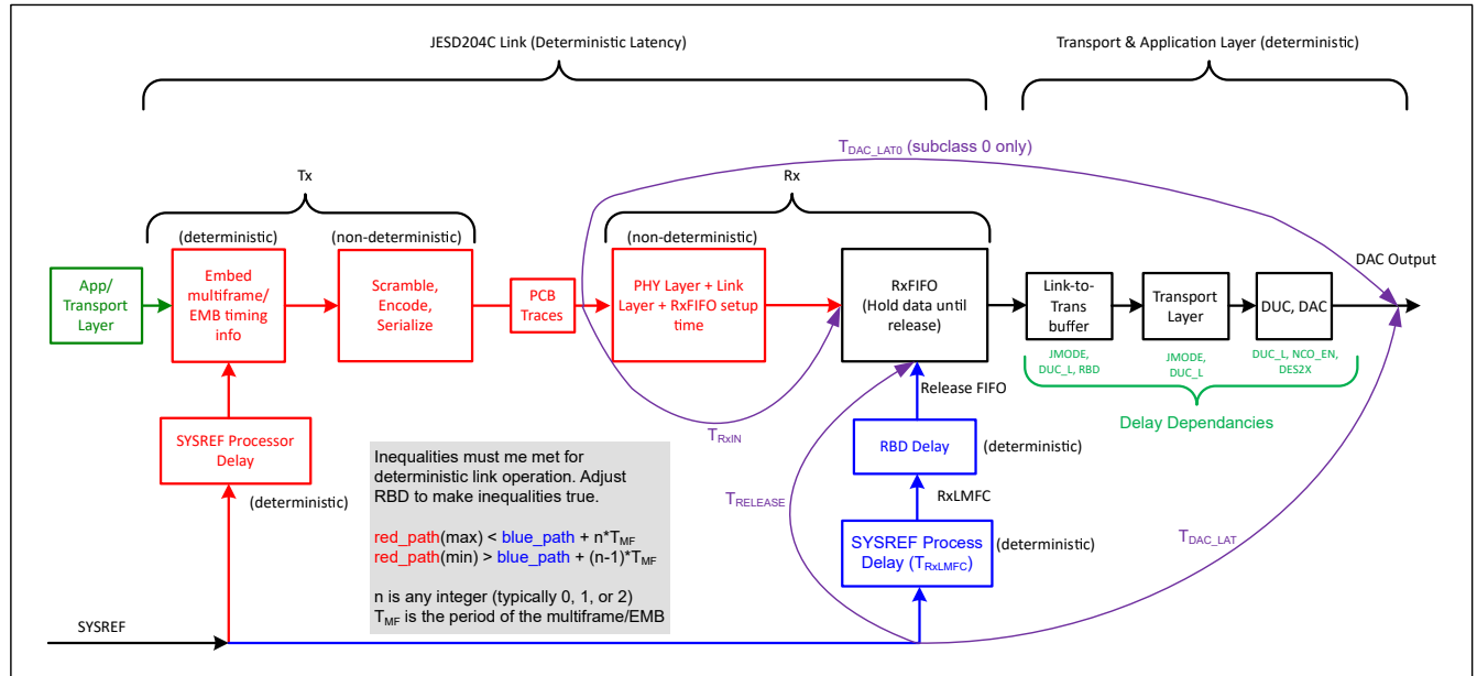
图 7-57. 器件延迟的定义
