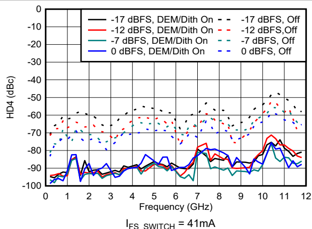
图 6-171. NRZ/RF 模式下 HD4 与频率和数字振幅间的关系
