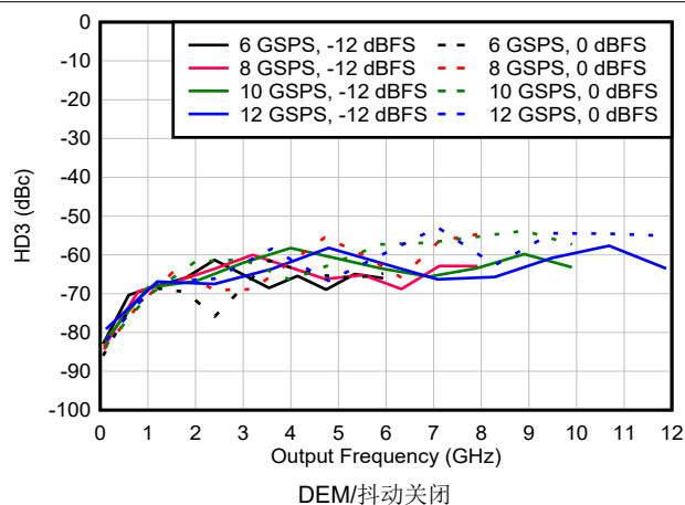
图 6-163. NRZ/RF 模式下 HD3 与频率和采样速率间的关系
