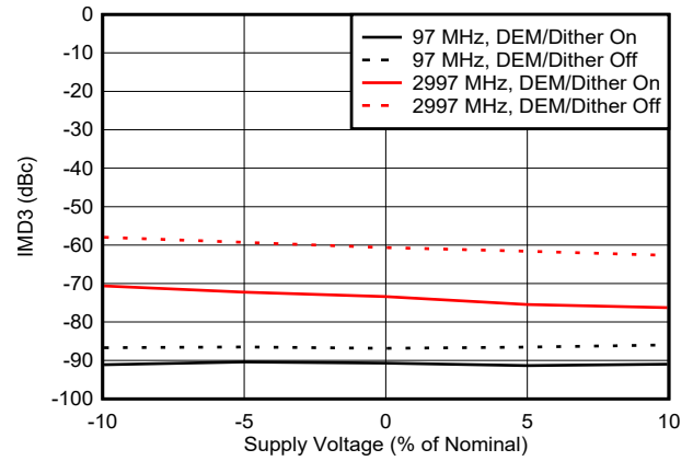
图 6-131. DES2XL 模式下 IMD3 与电压间的关系
