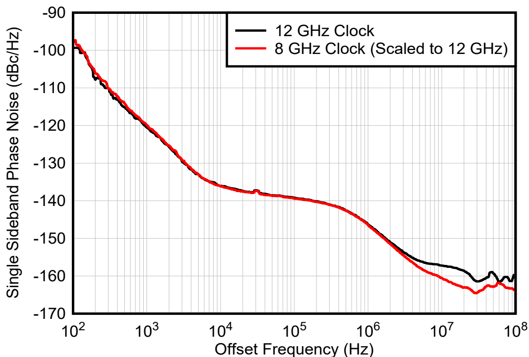
图 8-12. 8GHz 和 12GHz 时钟相位噪声
