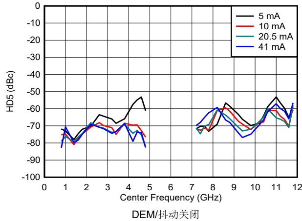
图 6-176. DES2X 模式下 HD5 与频率和输出电流间的关系
