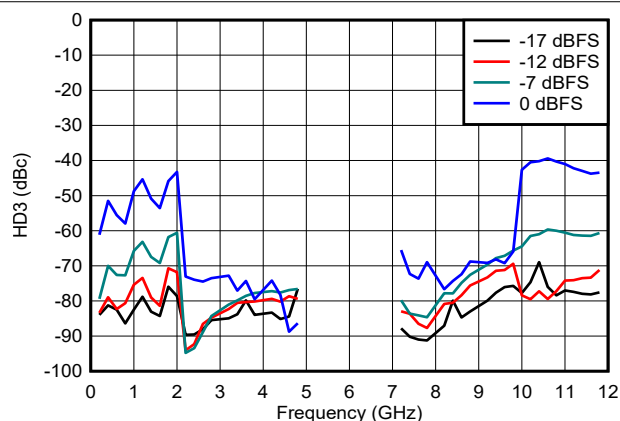
图 6-159. DES2X 模式下 HD3 与频率和数字振幅间的关系
