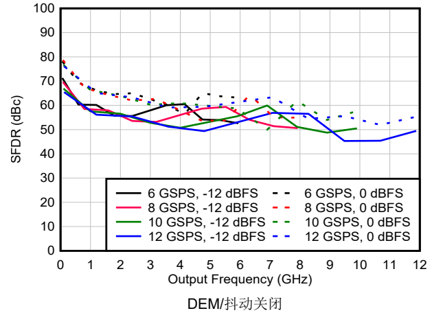
图 6-105. DES2X 模式下 SFDR 与频率和采样速率间的关系
