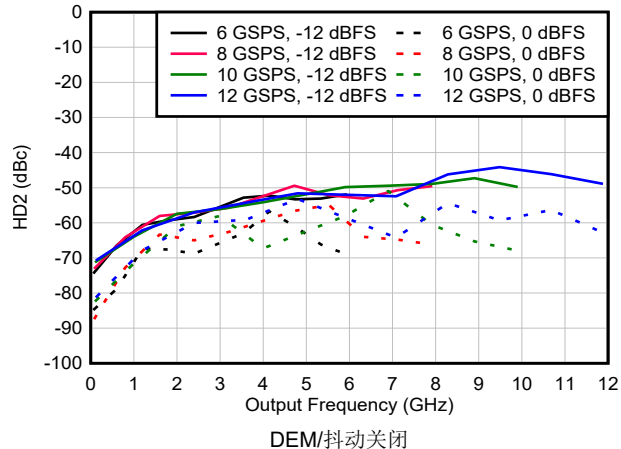
图 6-147. NRZ/RF 模式下 HD2 与频率和采样速率间的关系
