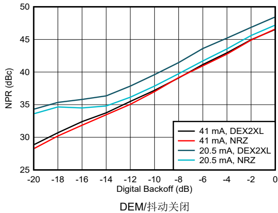
图 6-187. 噪声功率比与数字退避：第一奈奎斯特区域
