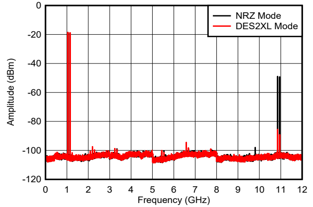
图 6-44. 双音， f_{\text{OUT}} = 1097\text{MHz} ，-6dBFS
