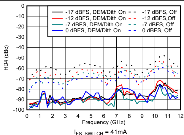
图 6-173. NRZ/RF 模式下 HD4 与频率和数字振幅间的关系
