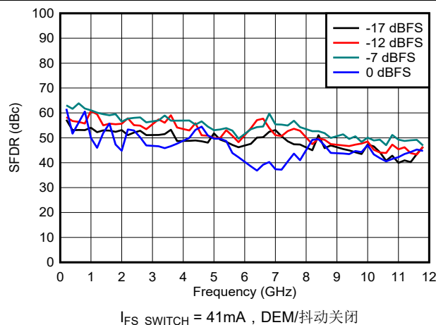
图 6-96. NRZ/RF 模式下 SFDR 与频率和数字振幅间的关系
