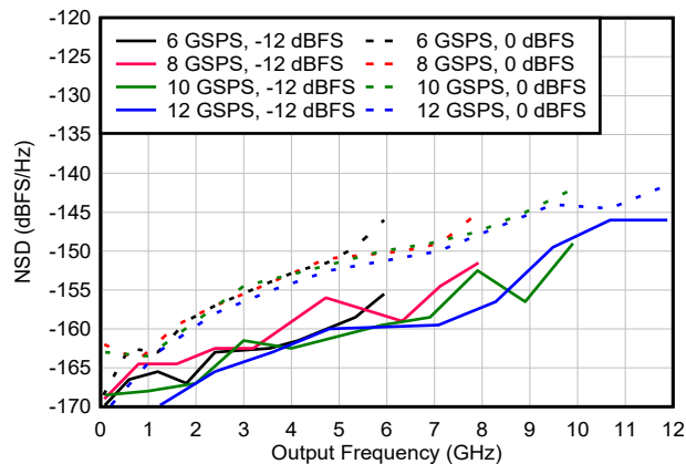
图 6-72. NSD 与输出频率和采样速率间的关系
