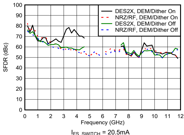
图 6-82. SFDR 与频率和模式间的关系
