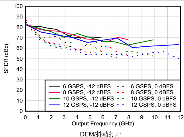
图 6-102. NRZ/RF 模式下 SFDR 与频率和采样速率间的关系
