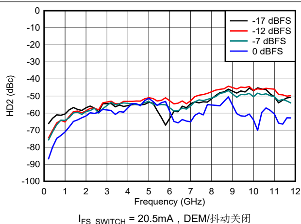
图 6-138. NRZ/RF 模式下 HD2 与频率和数字振幅间的关系
