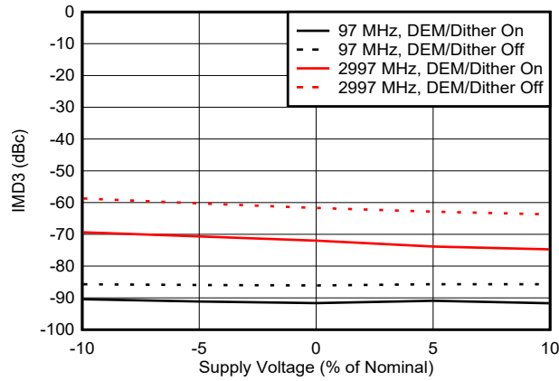
图 6-130. NRZ 模式下 IMD3 与电压间的关系
