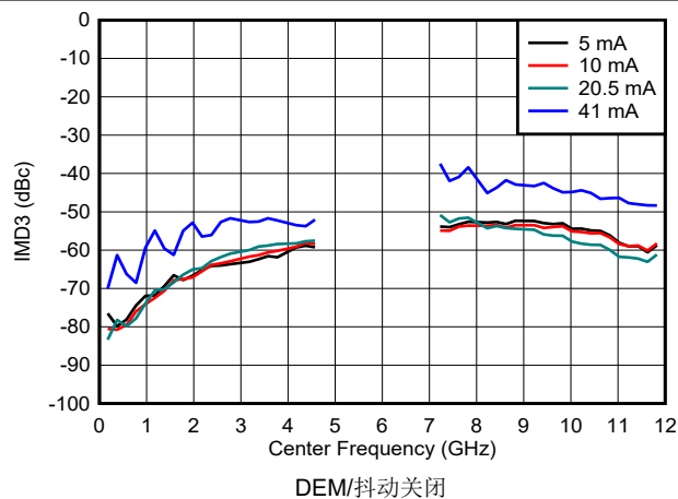
图 6-108. DES2X 模式下 IMD3 与频率和输出电流间的关系
