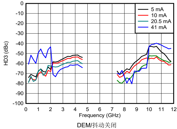
图 6-152. DES2X 模式下 HD3 与频率和输出电流间的关系
