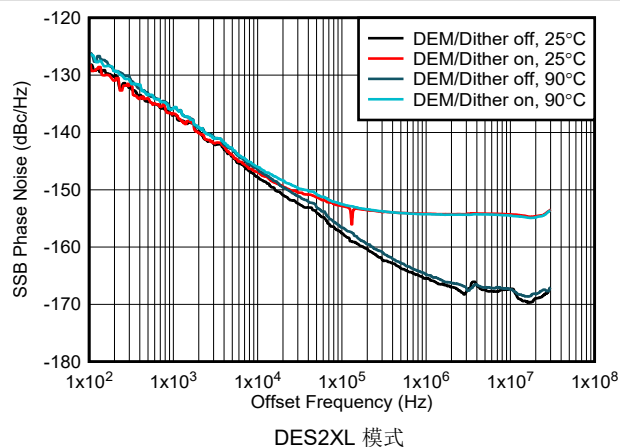
图 6-197. 1GHz 条件下相位噪声与偏移频率间的关系
