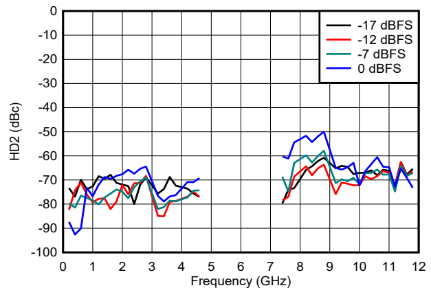
图 6-141. NRZ/RF 模式下 HD2 与频率和数字振幅间的关系
