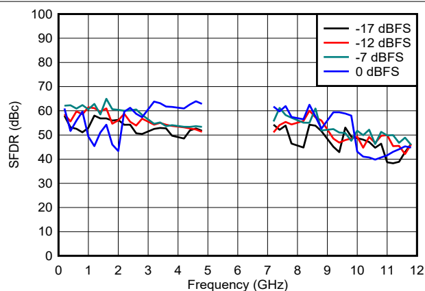
图 6-98. DES2X 模式下 SFDR 与频率和数字振幅间的关系
