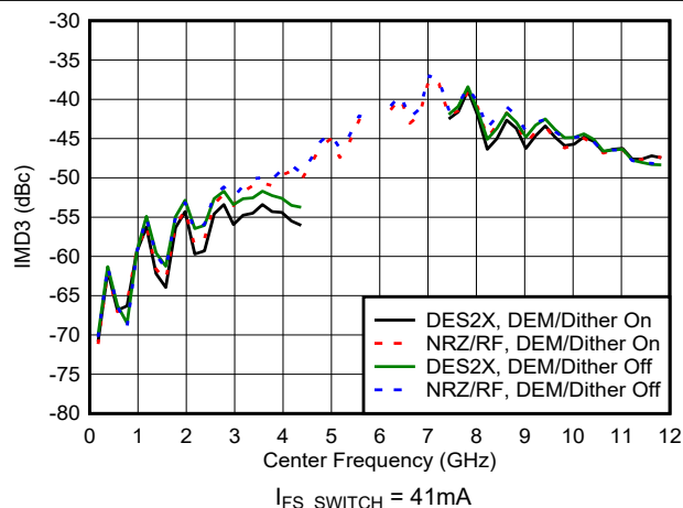
图 6-85. IMD3 与频率和模式间的关系
