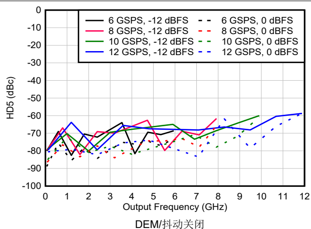
图 6-183. NRZ/RF 模式下 HD5 与频率和采样速率间的关系
