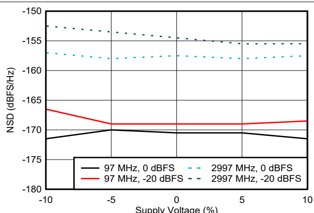
图 6-79. NSD 与电源电压间的关系
