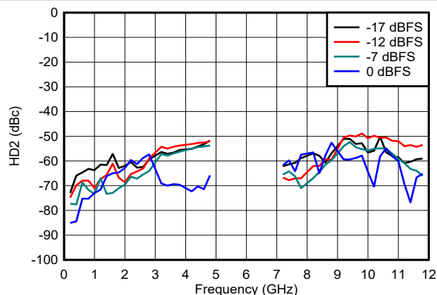
图 6-142. DES2X 模式下 HD2 与频率和数字振幅间的关系
