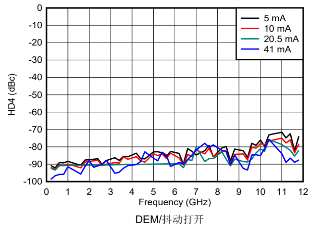
图 6-167. NRZ/RF 模式下 HD4 与频率和输出电流间的关系
