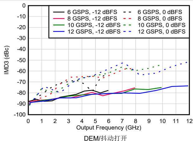
图 6-124. DES2X 模式下 IMD3 与频率和采样速率间的关系
