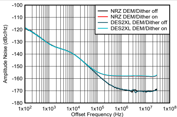
图 6-200. 1GHz 条件下振幅噪声与偏移频率间的关系
