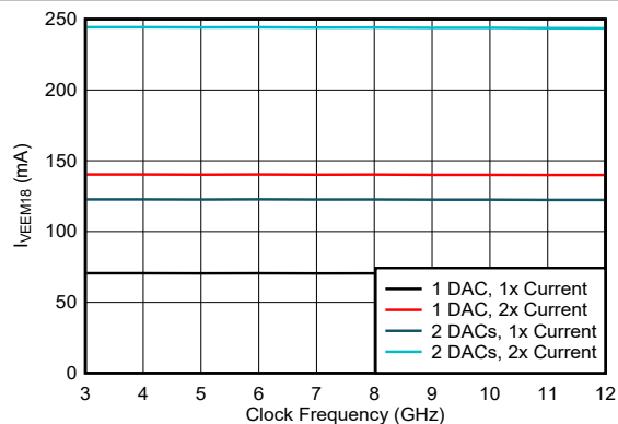
图 6-210. VEEM18 电流与时钟频率和 DAC 模式间的关系
