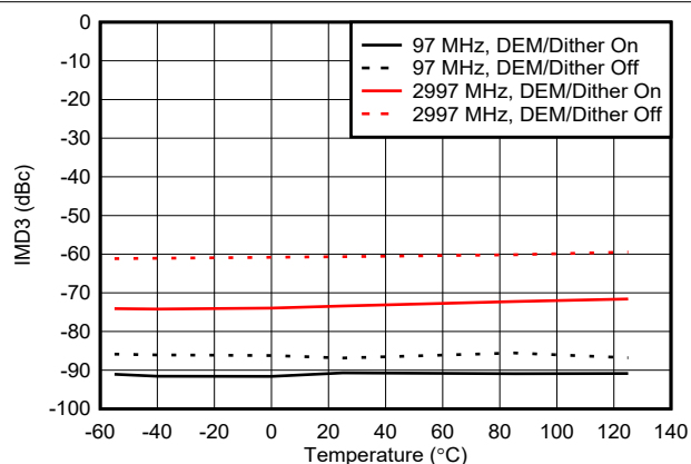
图 6-127. DES2XL 模式下 IMD3 与温度间的关系
