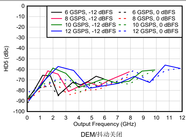
图 6-185. DES2X 模式下 HD5 与频率和采样速率间的关系
