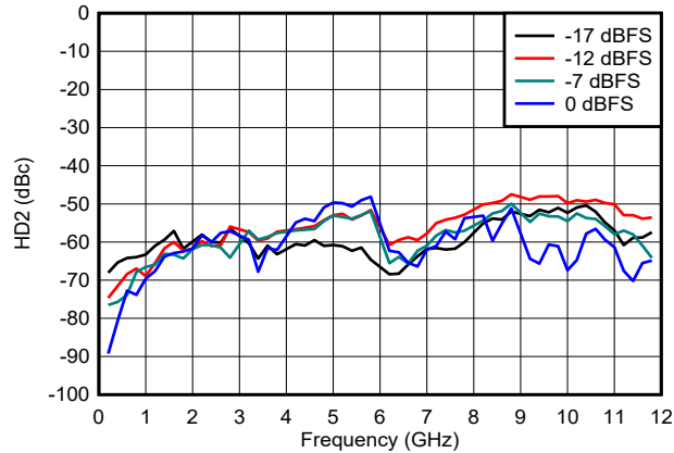
图 6-140. NRZ/RF 模式下 HD2 与频率和数字振幅间的关系
