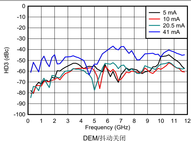
图 6-150. NRZ/RF 模式下 HD3 与频率和输出电流间的关系
