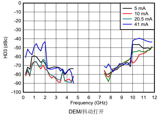
图 6-153. DES2X 模式下 HD3 与频率和输出电流间的关系
