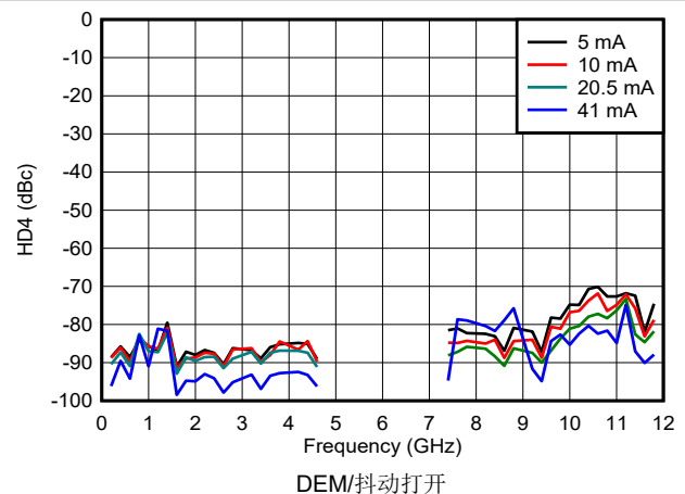
图 6-169. DES2X 模式下 HD4 与频率和输出电流间的关系
