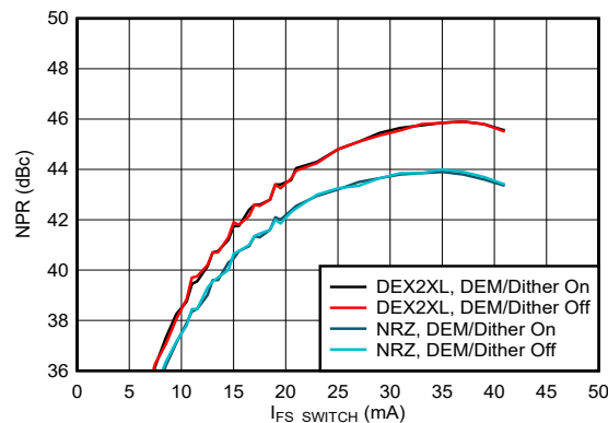
图 6-192. 电源抑制比与输出电流间的关系：第二个奈奎斯特区域
