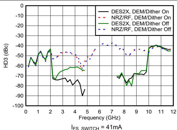
图 6-89. HD3 与频率和模式间的关系
