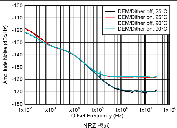
图 6-201. 1GHz 条件下振幅噪声与偏移频率和温度间的关系
