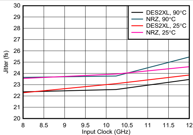
图 6-199. 抖动与输入时钟间的关系
