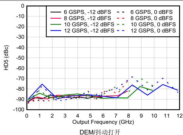
图 6-182. NRZ/RF 模式下 HD5 与频率和采样速率间的关系
