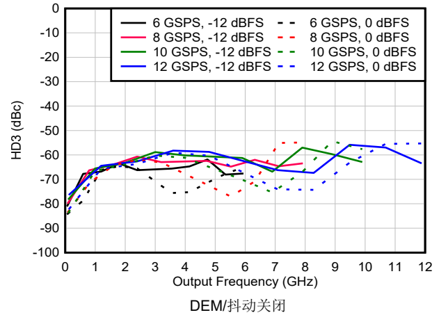
图 6-165. DES2X 模式下 HD3 与频率和采样速率间的关系
