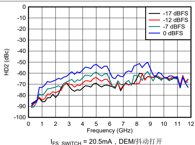
图 6-139. NRZ/RF 模式下 HD2 与频率和数字振幅间的关系
