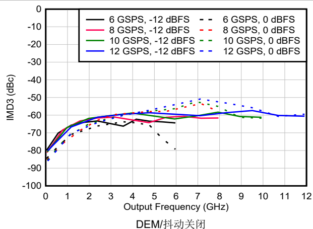
图 6-123. NRZ/RF 模式下 IMD3 与频率和采样速率间的关系
