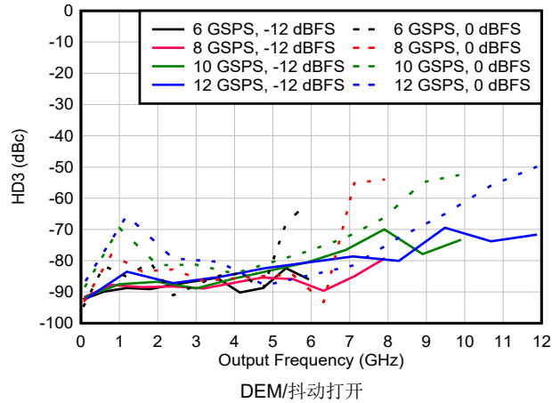
图 6-164. DES2X 模式下 HD3 与频率和采样速率间的关系
