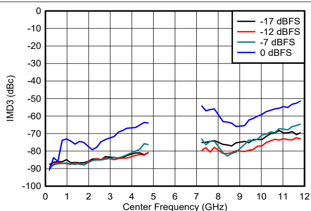
图 6-113. NRZ/RF 模式下 IMD3 与频率和数字振幅间的关系
