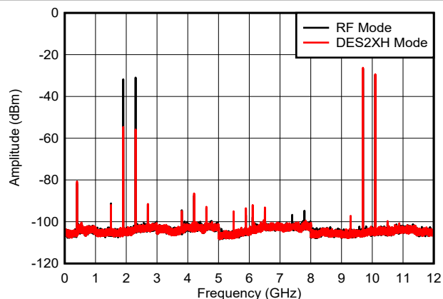
图 6-56. 双音， f_{\text{OUT}} = 9897\text{MHz} ，-6dBFS
