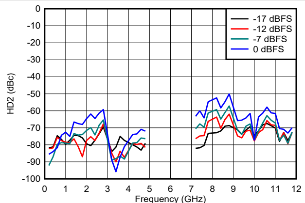
图 6-143. DES2X 模式下 HD2 与频率和数字振幅间的关系
