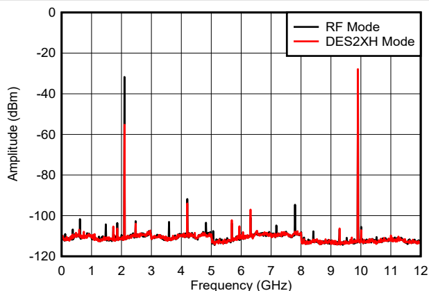
图 6-34. f_{\text{OUT}} = 9897\text{MHz} ，0dBFS
