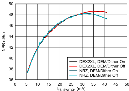
图 6-191. 电源抑制比与输出电流间的关系：第一奈奎斯特区域
