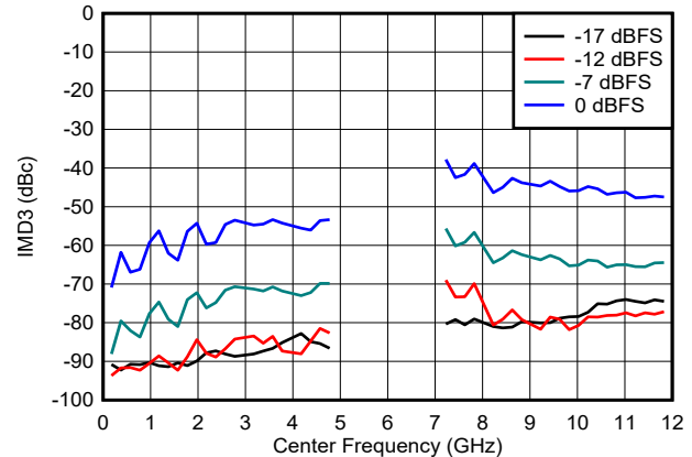
图 6-117. DES2X 模式下 IMD3 与频率和数字振幅间的关系
