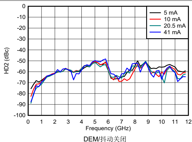
图 6-134. NRZ/RF 模式下 HD2 与频率和输出电流间的关系
