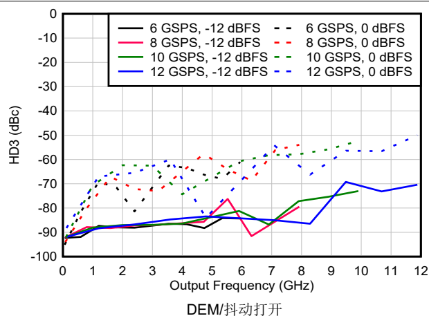
图 6-162. NRZ/RF 模式下 HD3 与频率和采样速率间的关系
