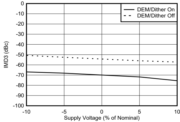
图 6-128. 9002MHz RF 模式下 IMD3 与电压间的关系
