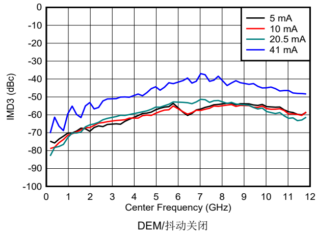
图 6-106. NRZ/RF 模式下 IMD3 与频率和输出电流间的关系
