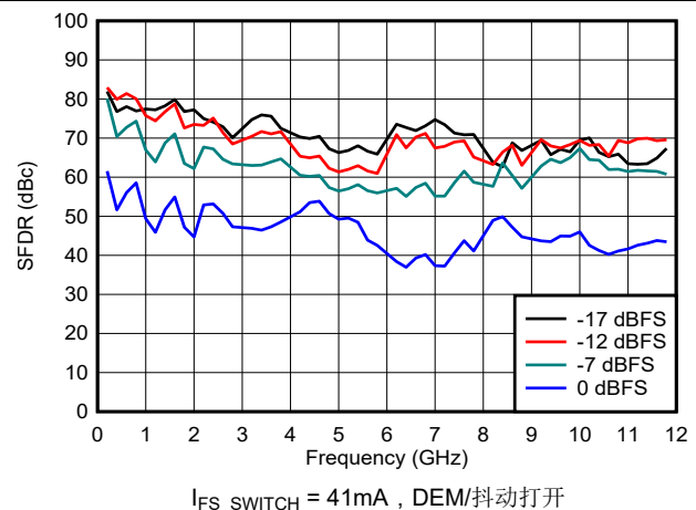
图 6-97. NRZ/RF 模式下 SFDR 与频率和数字振幅间的关系
