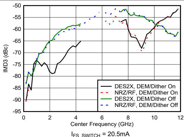
图 6-84. IMD3 与频率和模式间的关系
