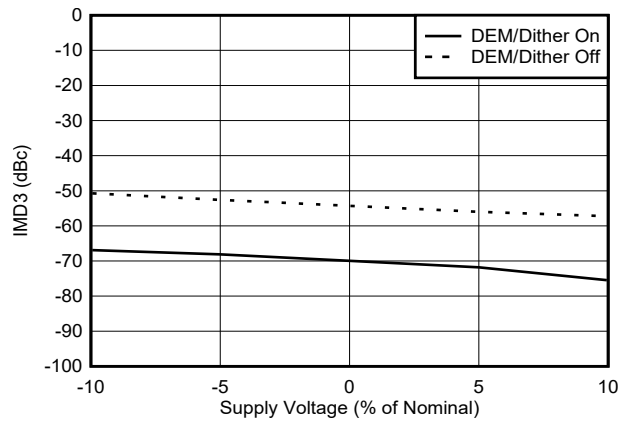
图 6-132. 9002MHz RF 模式下 IMD3 与电压间的关系
