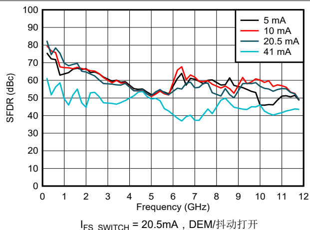
图 6-91. NRZ/RF 模式下 SFDR 与频率和输出电流间的关系
