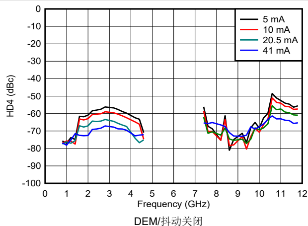
图 6-168. DES2X 模式下 HD4 与频率和输出电流间的关系
