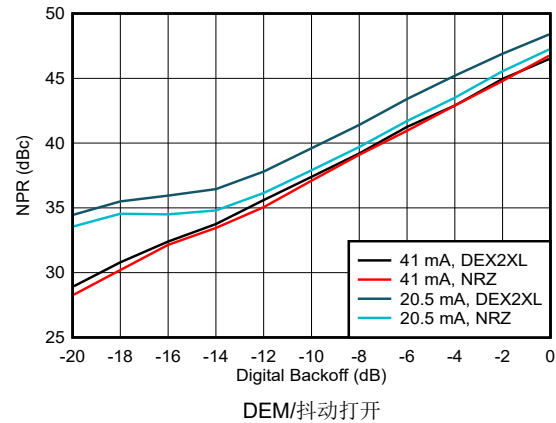
图 6-188. 噪声功率比与数字退避：第一奈奎斯特区域
