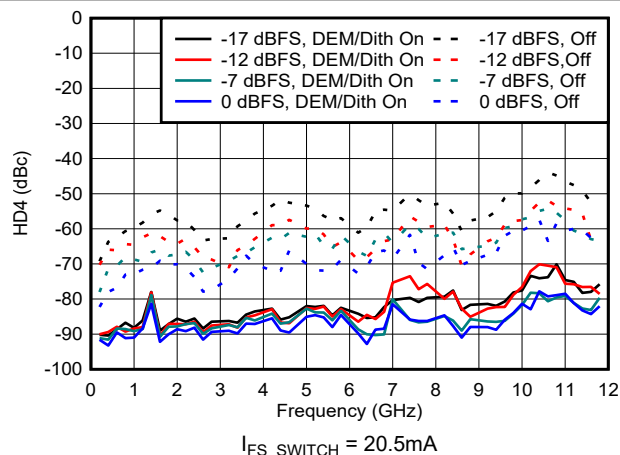
图 6-170. NRZ/RF 模式下 HD4 与频率和数字振幅间的关系
