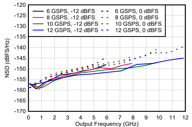
图 6-73. NSD 与输出频率和采样速率间的关系
