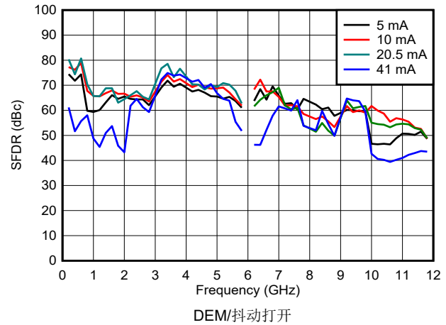
图 6-93. DES2X 模式下 SFDR 与频率和输出电流间的关系
