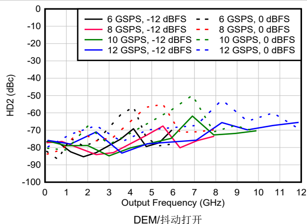
图 6-148. DES2X 模式下 HD2 与频率和采样速率间的关系
