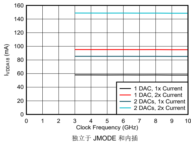
图 6-46. VDDA18 电流与时钟频率和 DAC 模式间的关系
