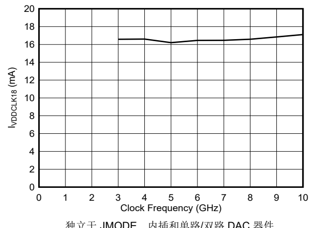
图 6-47. VDDCLK18 电流与时钟频率间的关系
