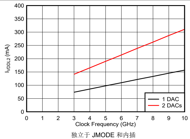
图 6-49. VDDLx 电流与时钟频率间的关系
