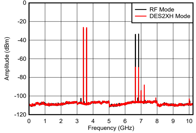
图 6-37. 双音， f_{\text{OUT}} = 3497\text{MHz} ，-12dBFS
