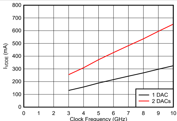
图 6-51. VDDE 电流与时钟频率间的关系
