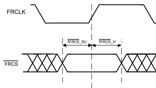
图 6-7. \overline{\text{FRCS}} 时序图
