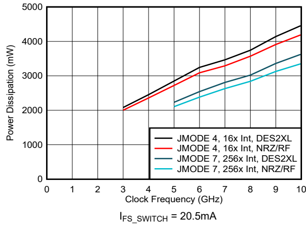
图 6-44. 功率损耗与时钟频率和数字模式间的关系
