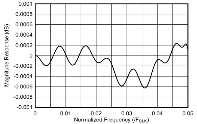
图 7-23. 8 倍内插滤波器通带响应
