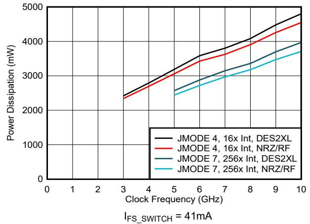
图 6-45. 功率损耗与时钟频率和数字模式间的关系
