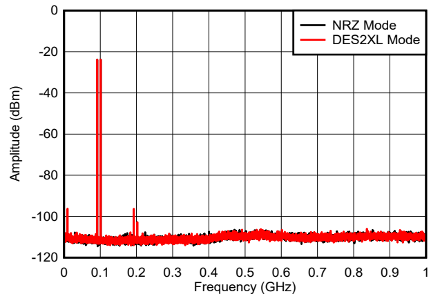
图 6-40. 双音， f_{\text{OUT}} = 97\text{MHz} ， -6\text{dBFS} ( 0\text{GHz} 至 1\text{GHz} )
