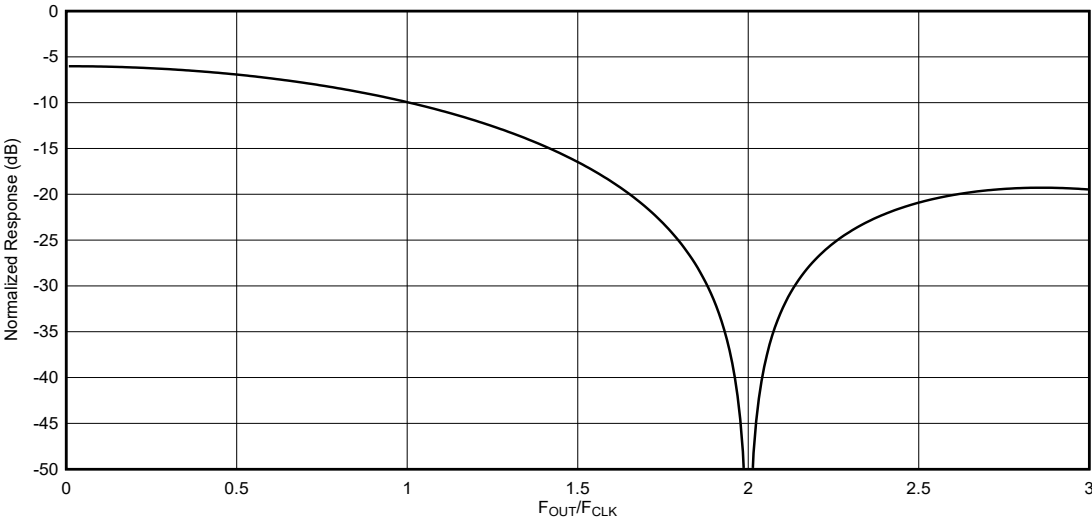
图 7-6. RTZ 模式输出频率响应
