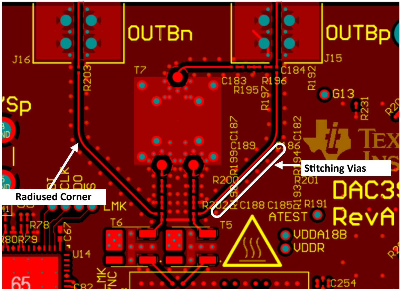
图 8-24. 高速信号布线旁边的半径角和拼接过孔
