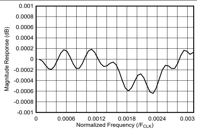
图 7-39. 128 倍内插滤波器通带响应
