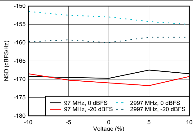
图 6-85. NSD 与电源电压间的关系
