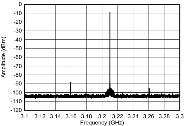
图 8-20. f_{OUT} = 3.211\text{GHz} 时的带内单音频谱
