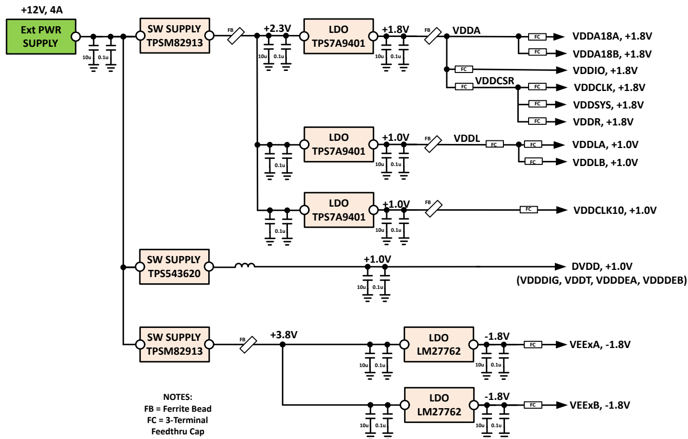
图 8-23. 推荐的电源方框图
