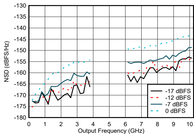
图 6-70. NSD 与输出频率和数字振幅间的关系
