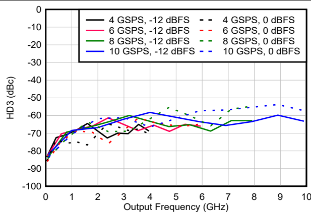
图 6-168. DES2X 模式下 HD3 与频率和数字振幅间的关系
