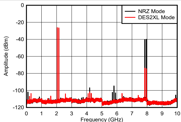
图 6-48. 双音， f_{\text{OUT}} = 2097\text{ MHz} ， -12\text{ dBFS}
