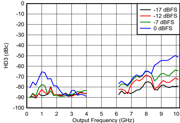
图 6-166. DES2X 模式下 HD3 与频率和数字振幅间的关系
