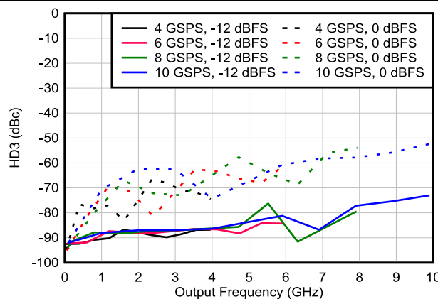
图 6-167. DES2X 模式下 HD3 与频率和数字振幅间的关系
