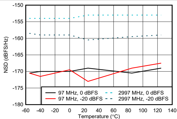
图 6-81. NSD 与温度间的关系
