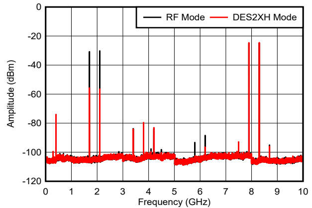
图 6-56. 双音， f_{\text{OUT}} = 8097\text{ MHz} ，-6dBFS
