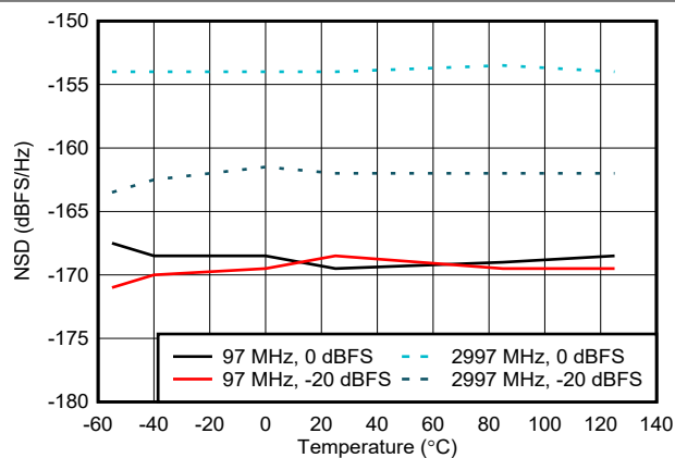
图 6-83. NSD 与温度间的关系
