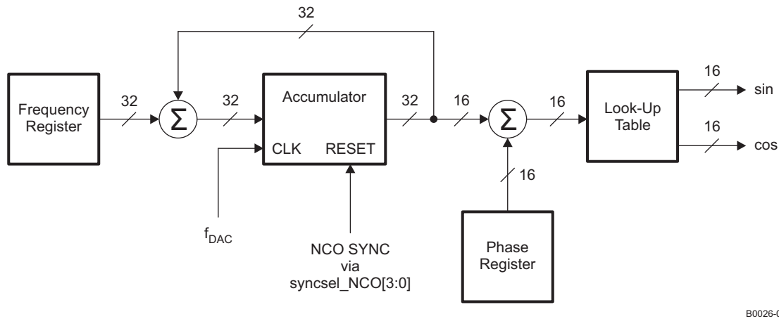
图 70. NCO Block Diagram
