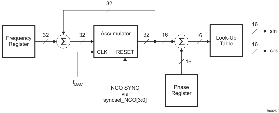
图 6-22. NCO Block Diagram
