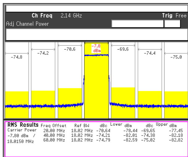
图 7-2. 20MHz TM1.1 LTE Carrier at 2.14GHz
