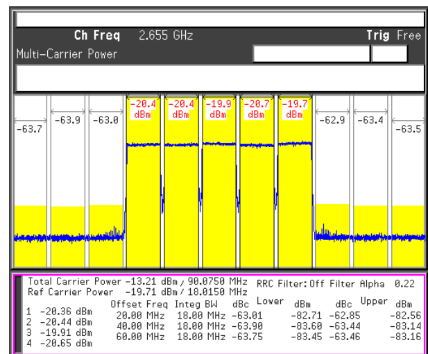
图 7-8. 5x20MHz TM1.1 LTE Carrier at 2.655GHz
