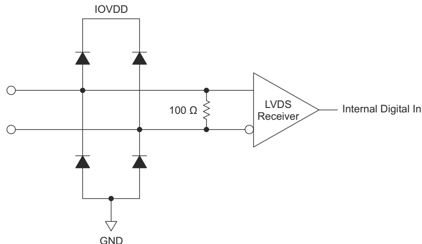
图 6-33. D[15:0]P/N, DATACLKP/N, FRAMEP/N, SYNCN/P and PARITYTYP/N LVDS Input Configuration
