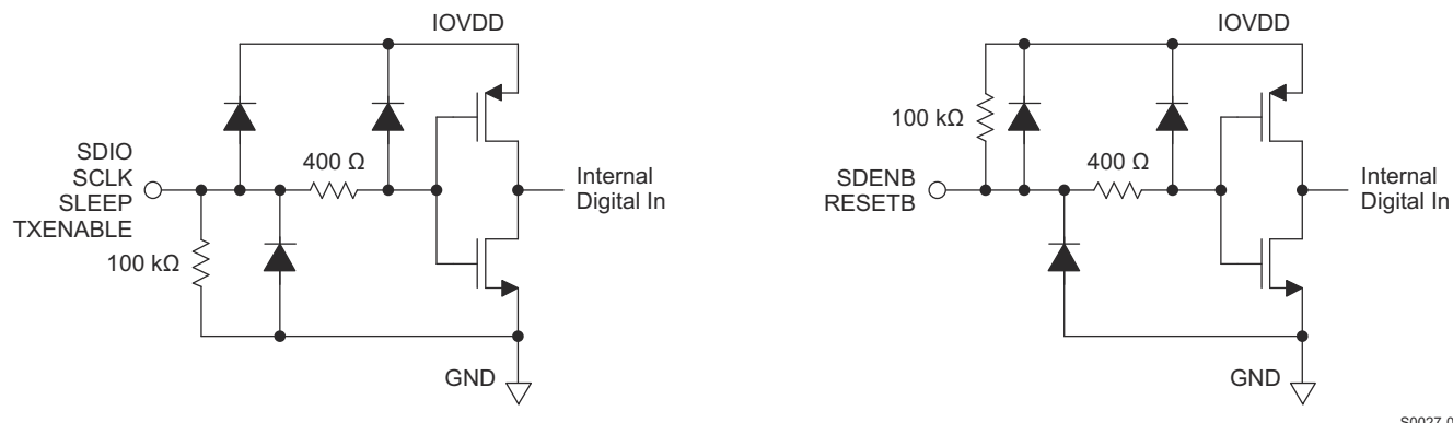
图 6-36. CMOS Digital Equivalent Input
