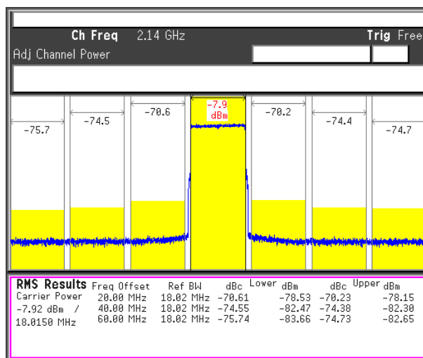
图 7-3. 20MHz TM1.1 LTE Carrier at 2.14GHz
