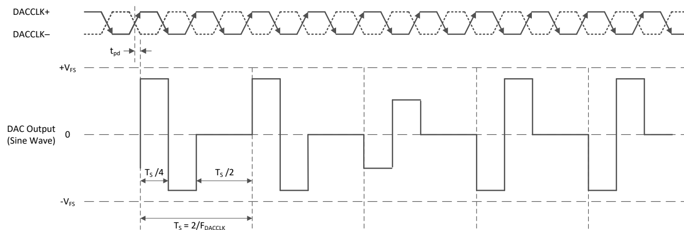
图 7-7. 2xRF Mode Timing Diagram
