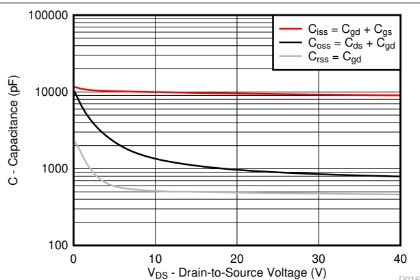
图 4-11. MOSFET Capacitance
