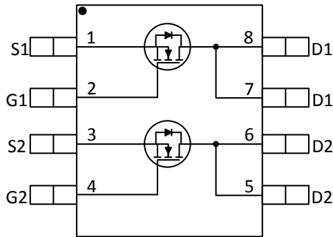
图 3-1. 顶视图
