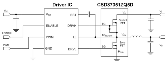
典型电路
