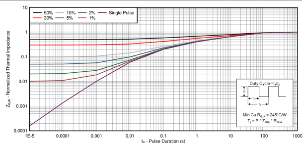
图 5-1. Transient Thermal Impedance
