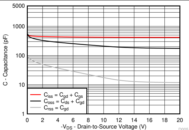
图 5-5. Capacitance
