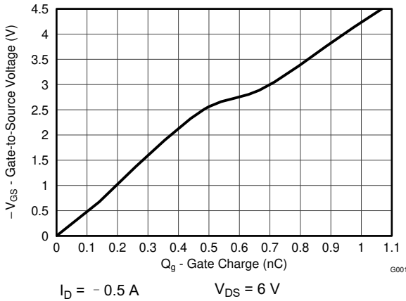
图 5-4. Gate Charge
