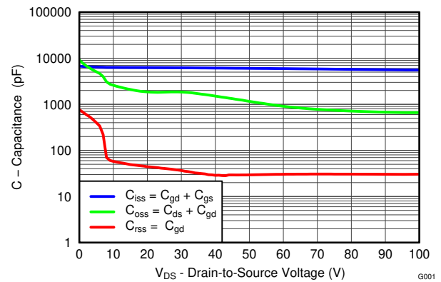
图 4-5. Capacitance
