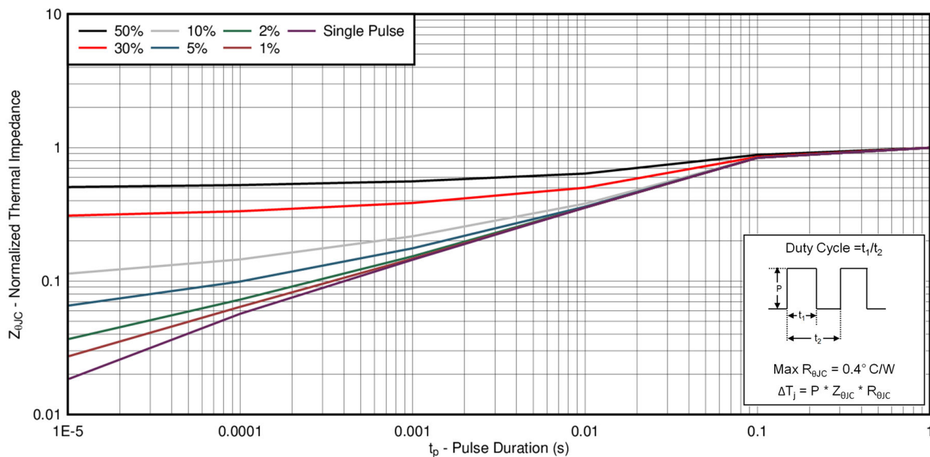
图 3-1. 瞬态热阻抗
