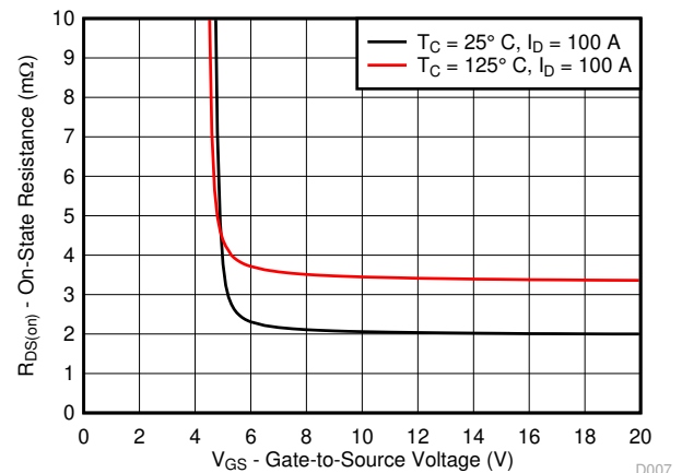
图 3-7. 导通电阻与栅源电压的关系
