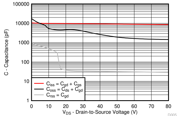
图 3-5. 电容
