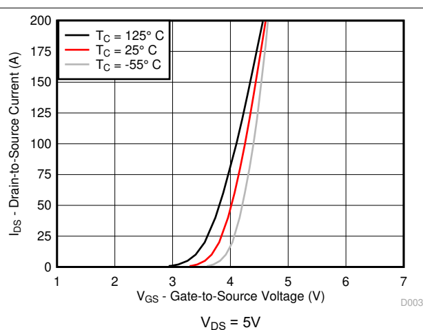
图 4-3. 传输特性
