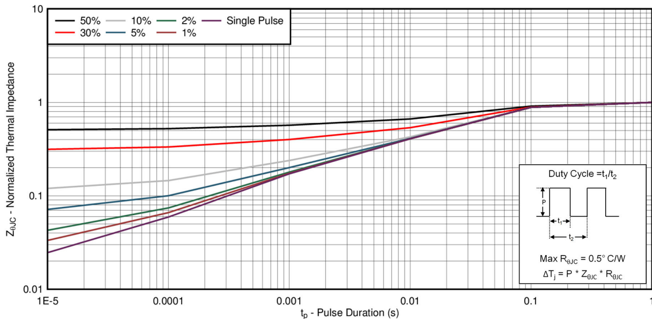
图 4-1. 瞬态热阻抗
