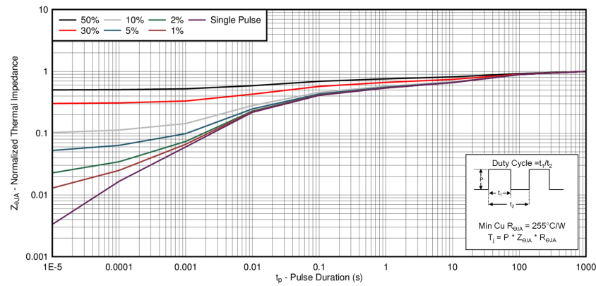
图 5-3. Transient Thermal Impedance
