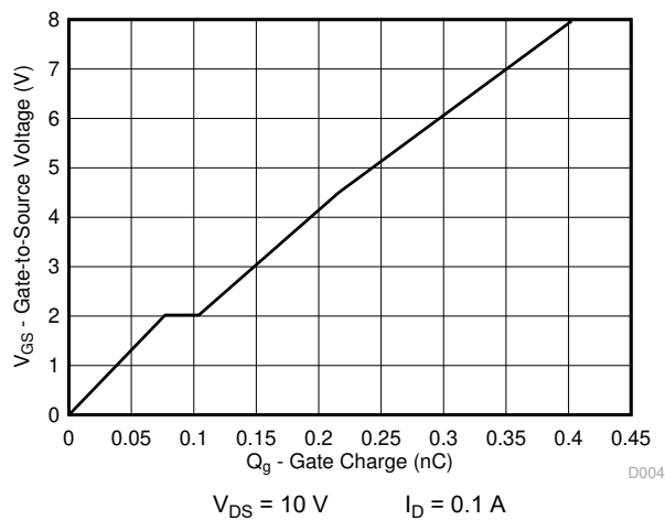
图 5-4. Gate Charge
