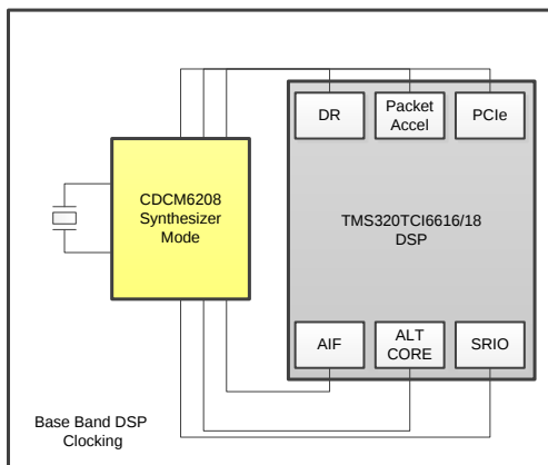
简化原理图
