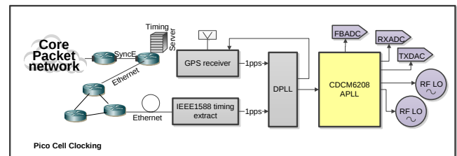
简化电路原理图
