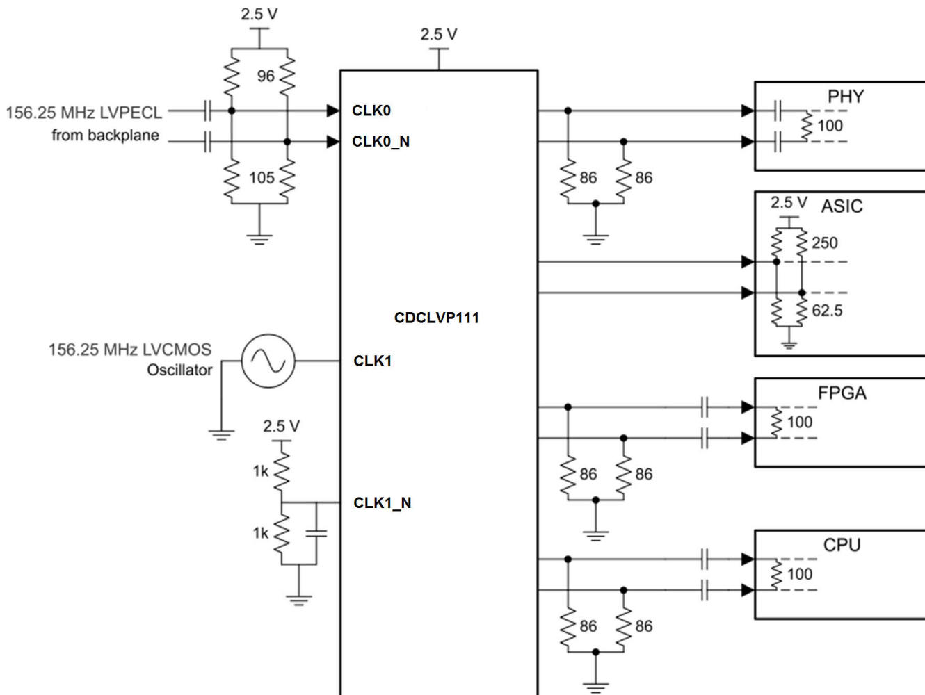
图 8-1. CDCLVP111-SEP 方框图
