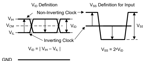
图 6-1. 差分输入信号的不同定义
