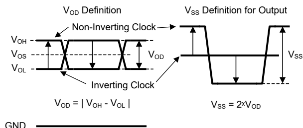
图 6-2. 差分输出信号的不同定义
