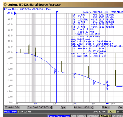
图 8-17. CDCLVP111-SEP 输出相位噪声, 13fs、2.4GHz (12kHz 至 20MHz)
