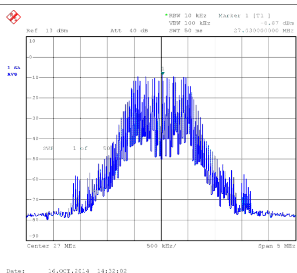
图 9-9. SSC 开启时的输出频谱，2% 中心
