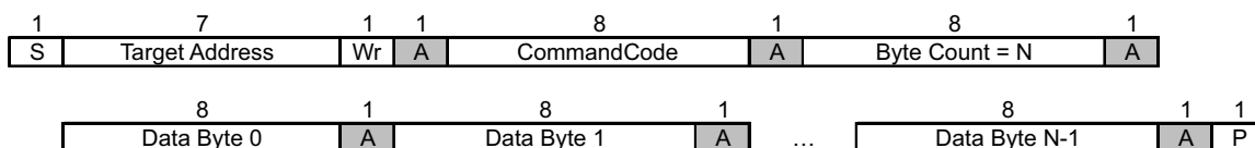
图 7-7. 块写入编程
