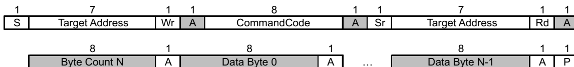
图 7-8. 块读取协议
