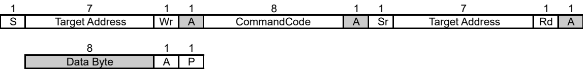
图 7-5. Byte Read Protocol
