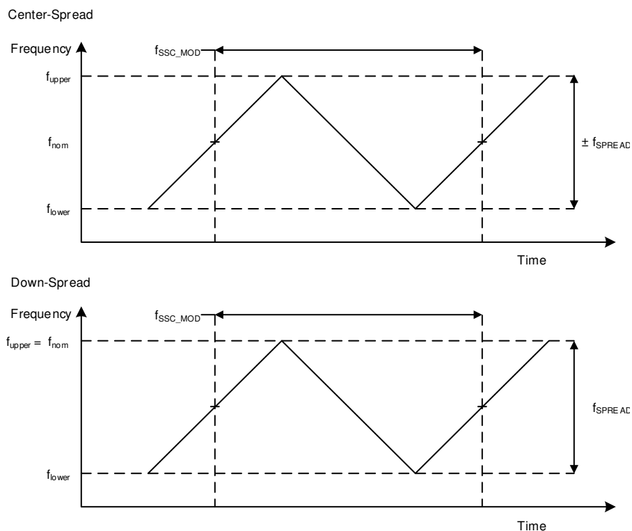
图 10-3. 展频时钟
