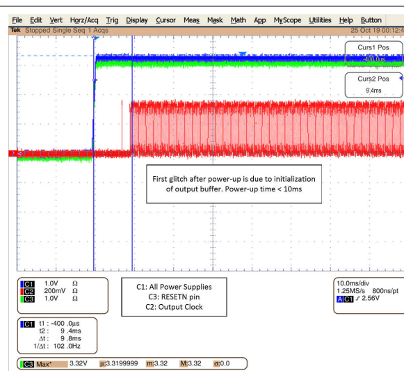
图 8-6. 所有电源 = 3.3V , VDD 斜坡时间 = 1ms
