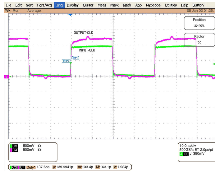
图 10-2. LVCMOS 输出的外部零延迟模式下的输入/输出对齐
