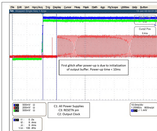
图 8-5. 所有电源 = 1.8V , VDD 斜坡时间 = 1ms
