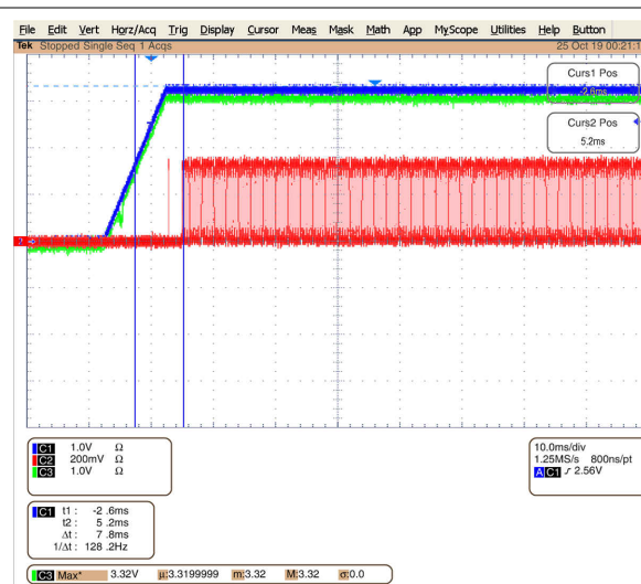
图 8-8. 所有电源 = 3.3V , VDD 斜坡时间 = 10ms
