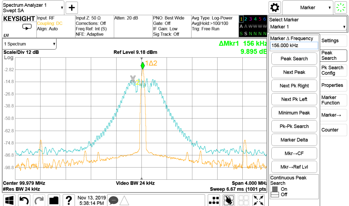
图 7-5. 100MHz，带 \pm 0.25\% 中心展频，有跟踪和无跟踪
