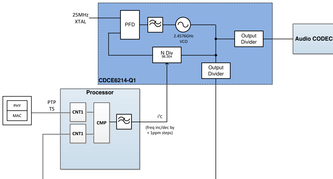
图 8-2. 使用 CDCE6214-Q1 的 eAVB 系统方框图
