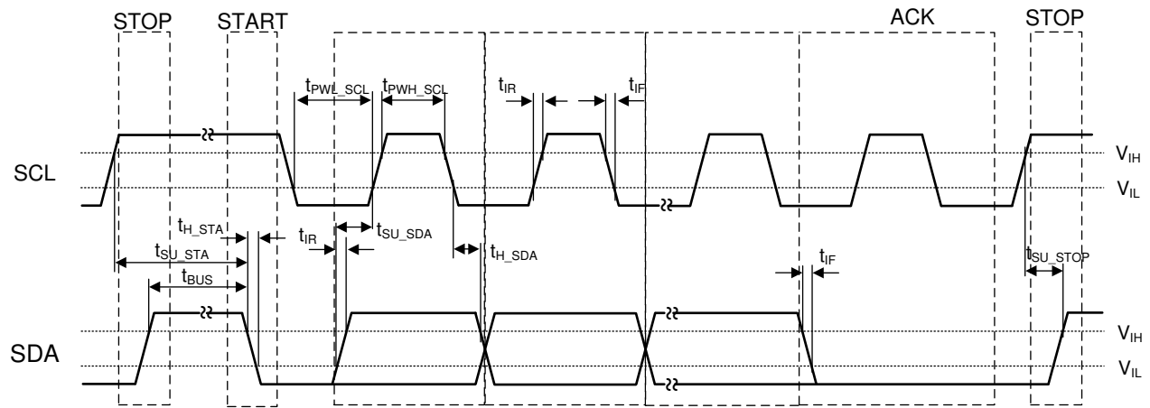
图 6-7. I²C 时序
