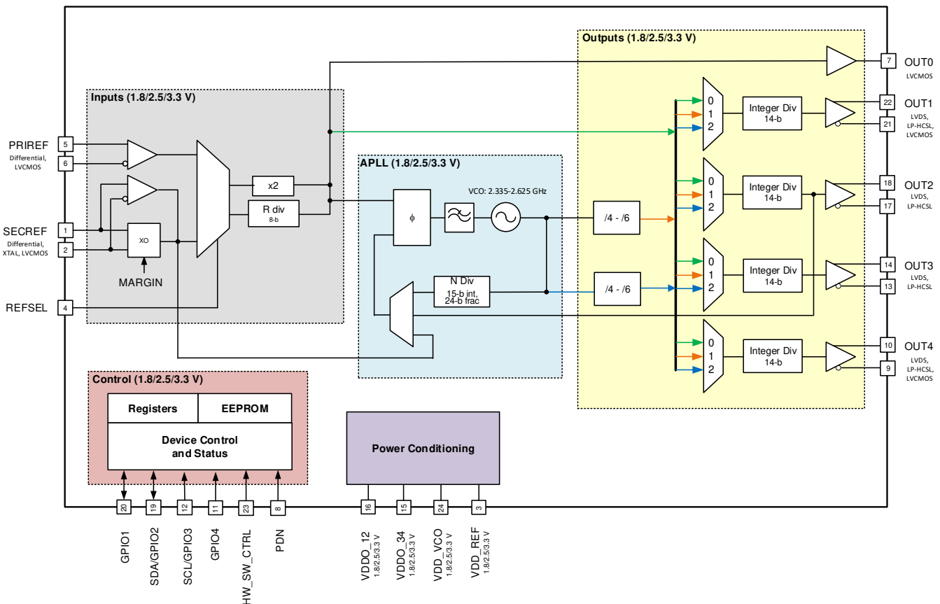
图 7-1. CDCE6214-Q1 具有两个输入、一个分数 N PLL 和四个输出的时钟发生器
