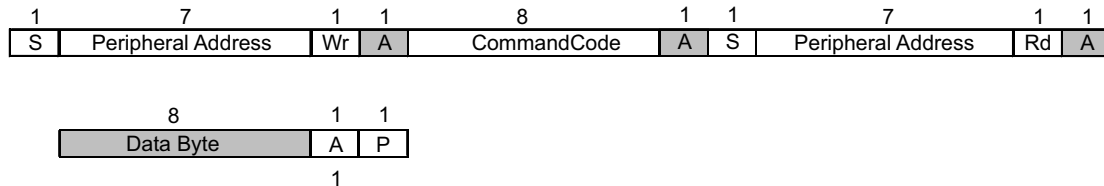
图 8-4. Byte Read Protocol
