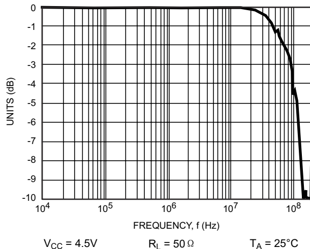
图 14-2. 典型开关频率响应
