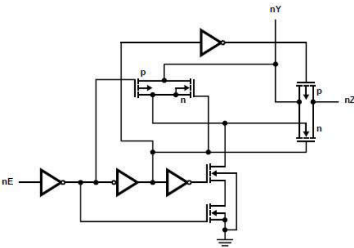
图 16-2. Logic Diagram
