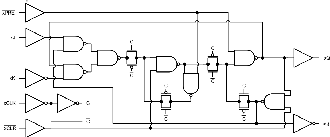
功能图
