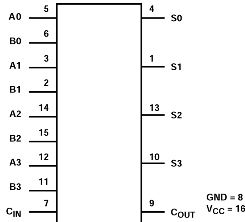
功能方框图
