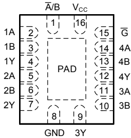
图 4-2. CD74AC157 BQB 封装 (顶视图)
