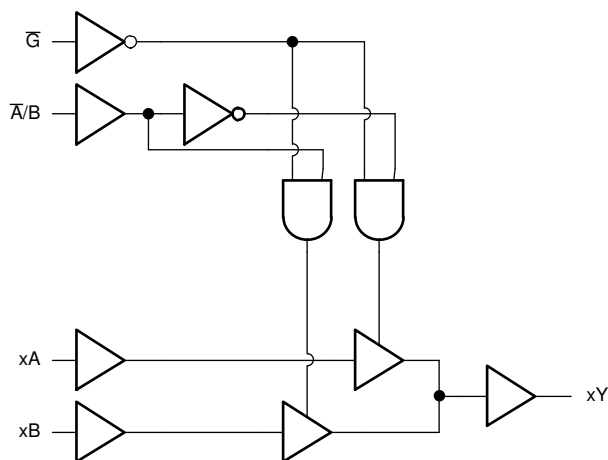
逻辑图
