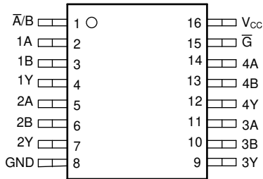
图 4-3. CD74AC157 D、N 封装 (顶视图)
