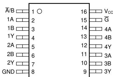
图 4-1. CD54AC157 J 封装 ( 顶视图 )
