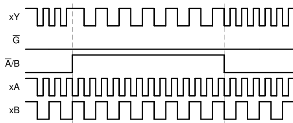
图 8-2. 应用时序图
