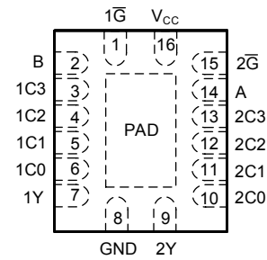
图 3-2. CD74AC153 BQB 封装；16 引脚 WQFN（顶视图）
