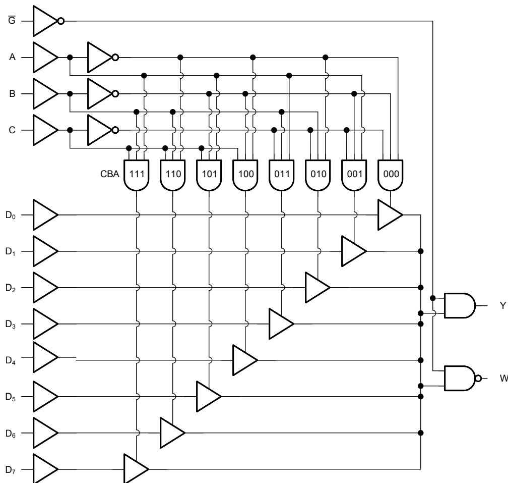
图 6-1. CD74AC151 的逻辑图 (正逻辑)
