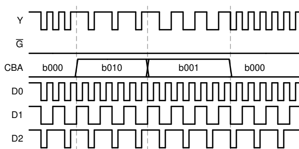
图 7-2. 应用时序图
