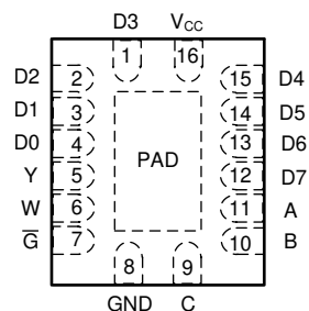
图 3-2. BQB 封装，16 引脚 WQFN（透明顶视图）
