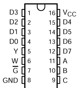
图 3-1. D、N 或 PW 封装；16 引脚 SOIC、PDIP 或 TSSOP（顶视图）
