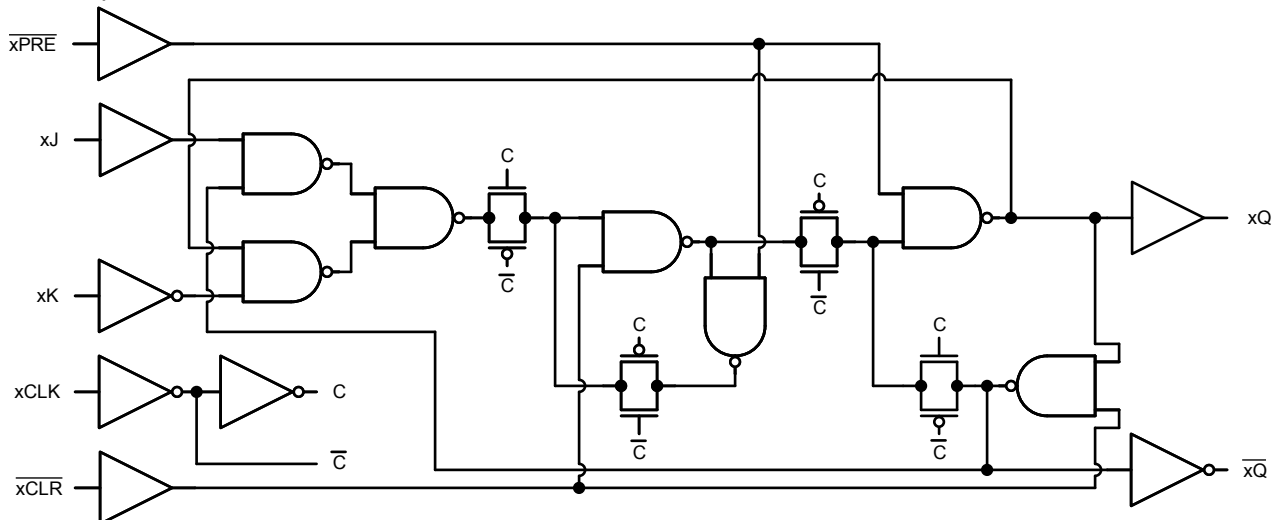
功能图
