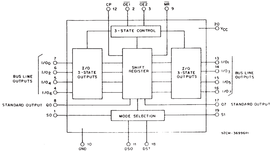
功能图
