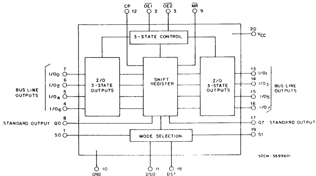
图 6-1. 功能图
