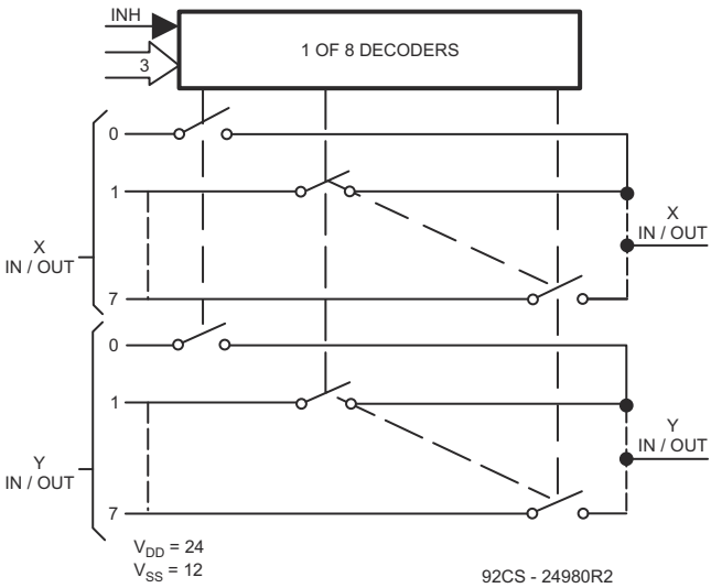
图 7-2. CD4097
