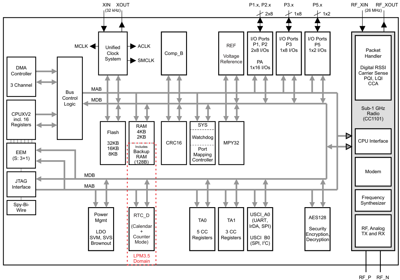
图 1-3 展示了 CC430F512x 器件的功能方框图。
