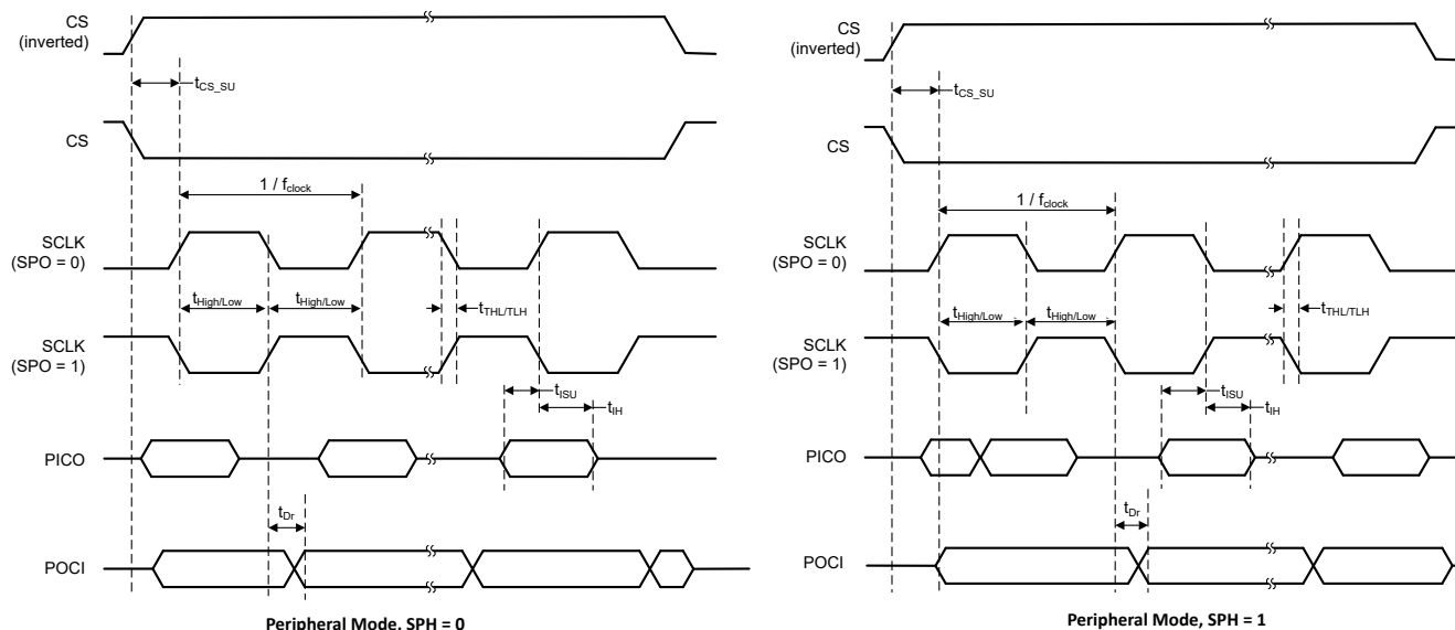
图 6-5. SPI 时序
