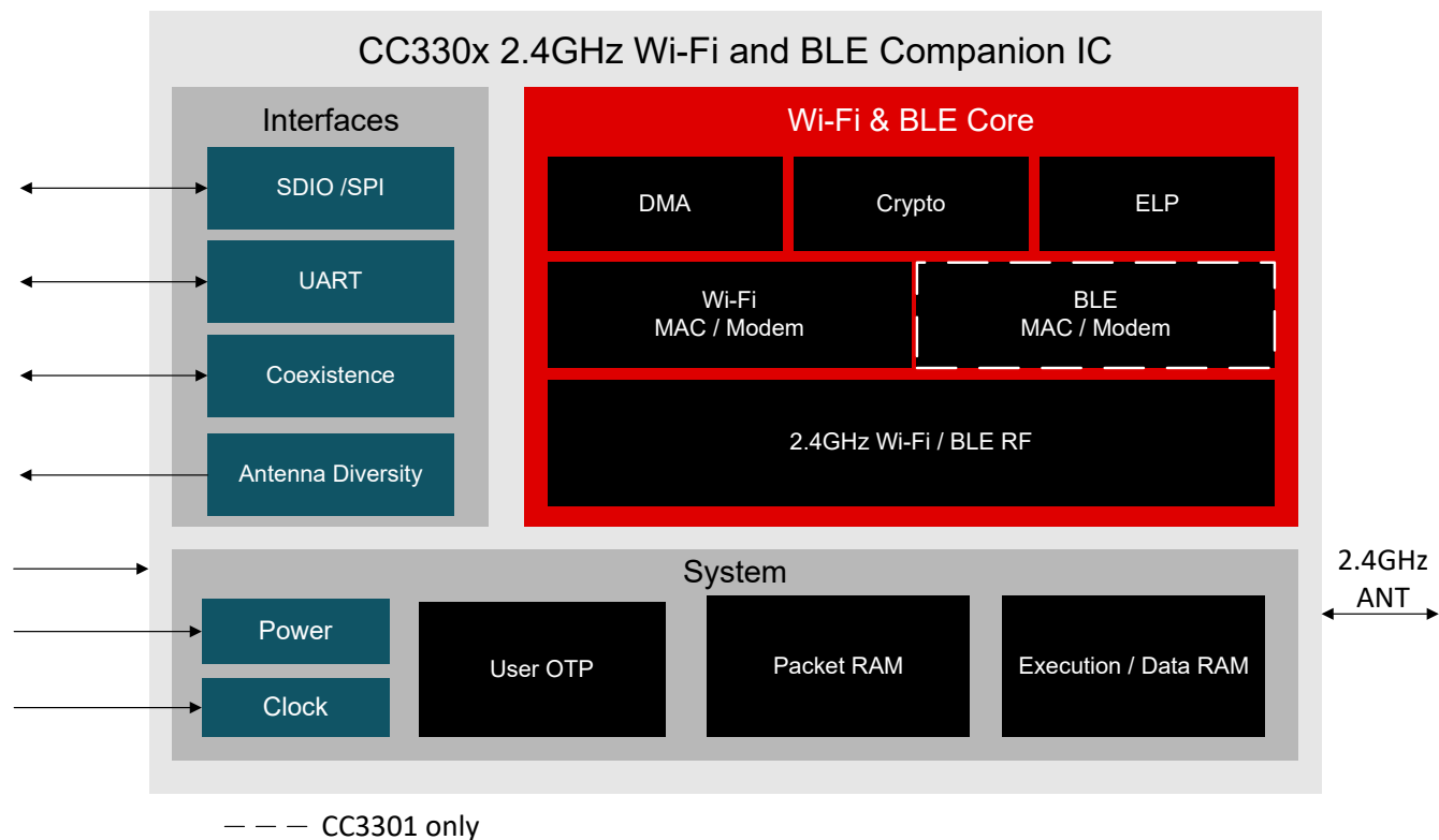
图 4-1. CC3301 系统简图
