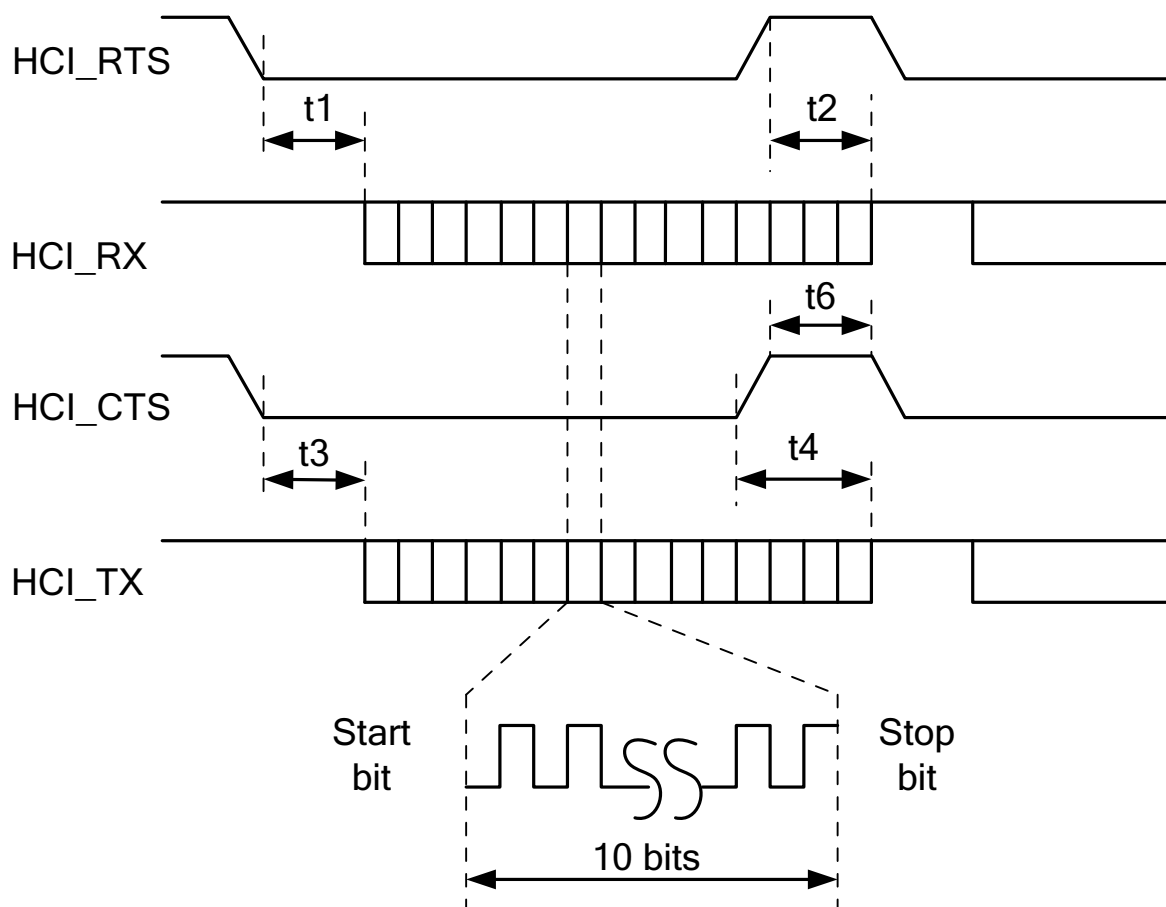
图 6-6. UART 时序图
