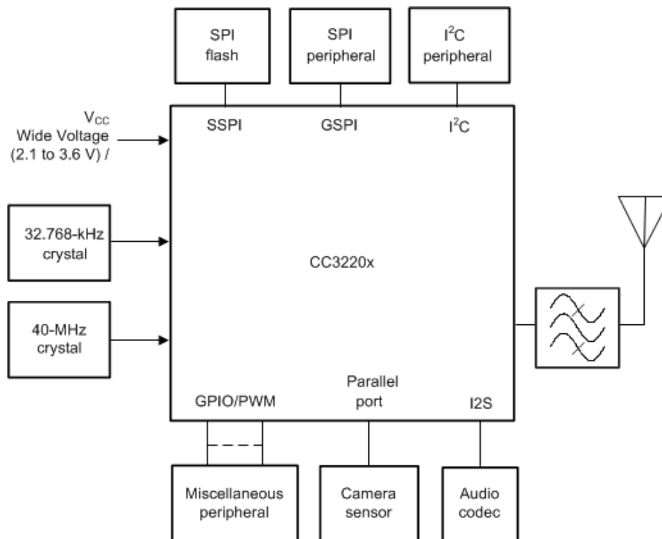
图 4-1. 功能模块图
