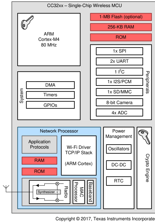
图 4-4. CC3220x 硬件概述
