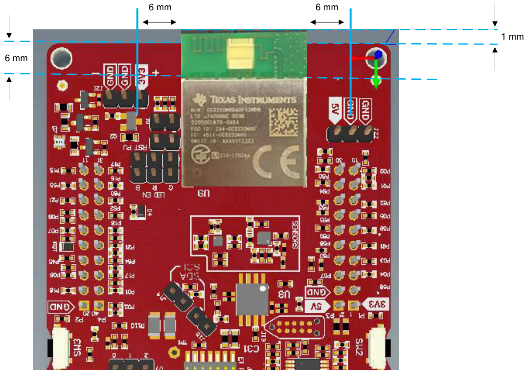
图 10-6. CC3220MODAx Layout Guidelines
