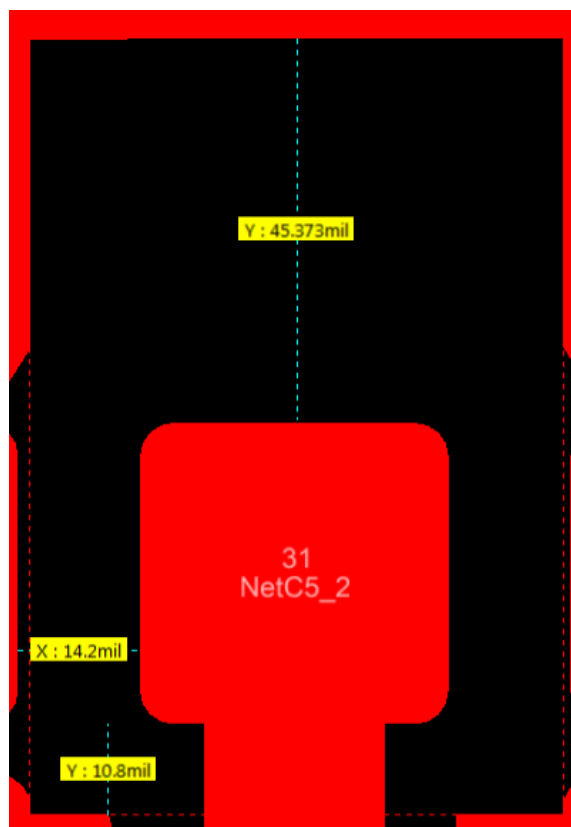
图 10-3. Top Layer Copper Pullback on RF Pads
